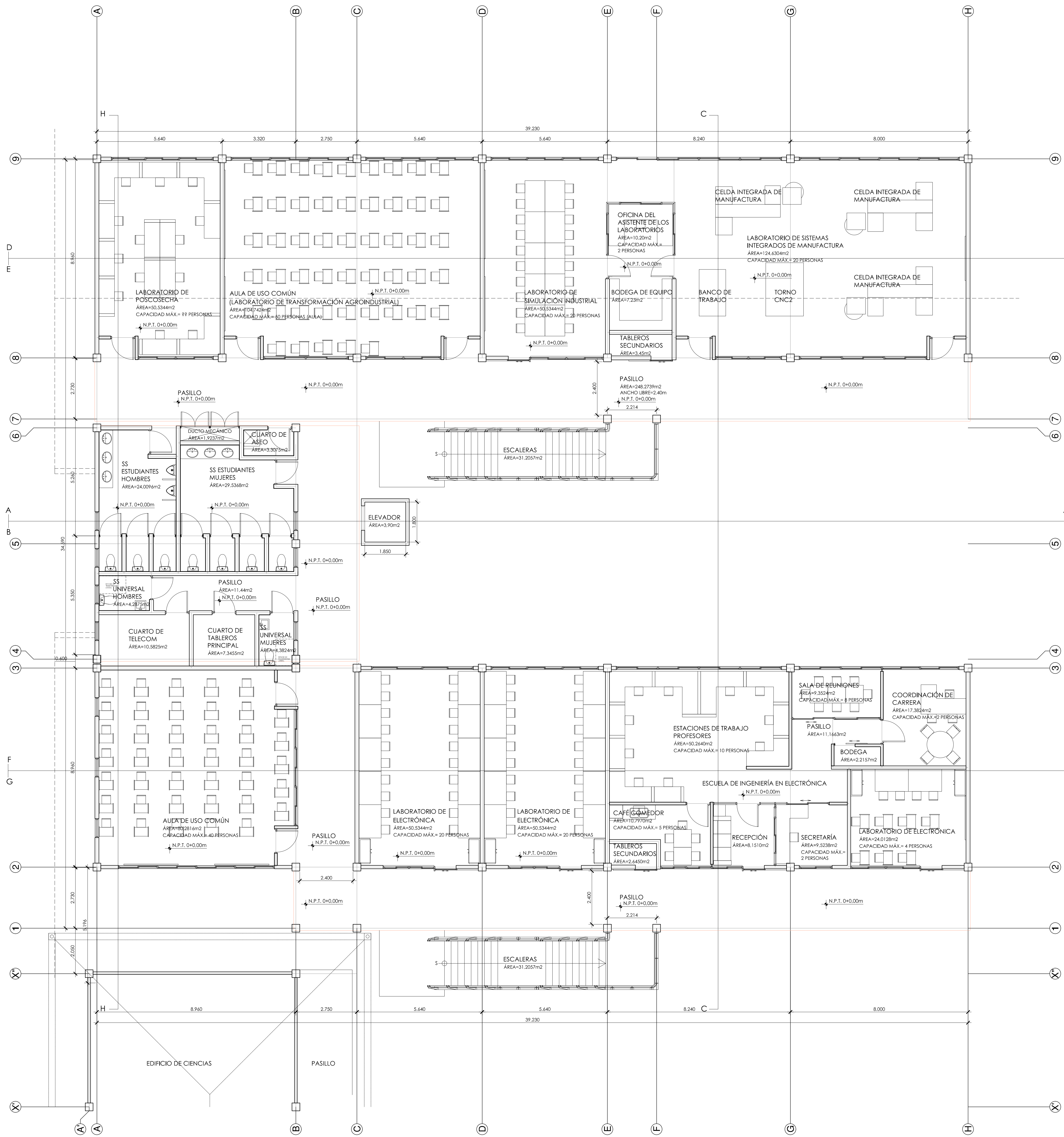
PLANTA ARQUITECTÓNICA NIVEL 1 escala 1: 75
