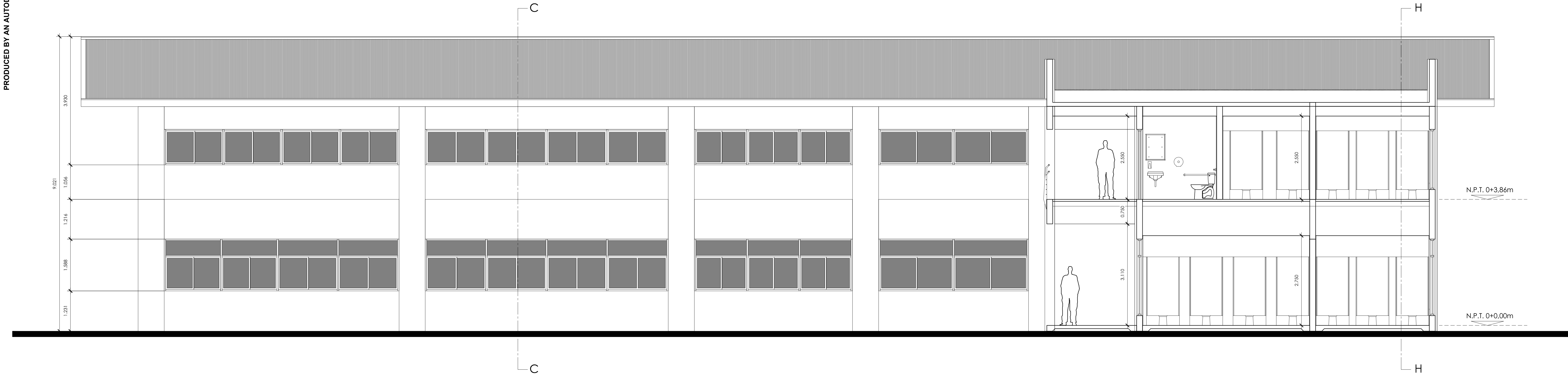
CORTE BB escala 1: 50
