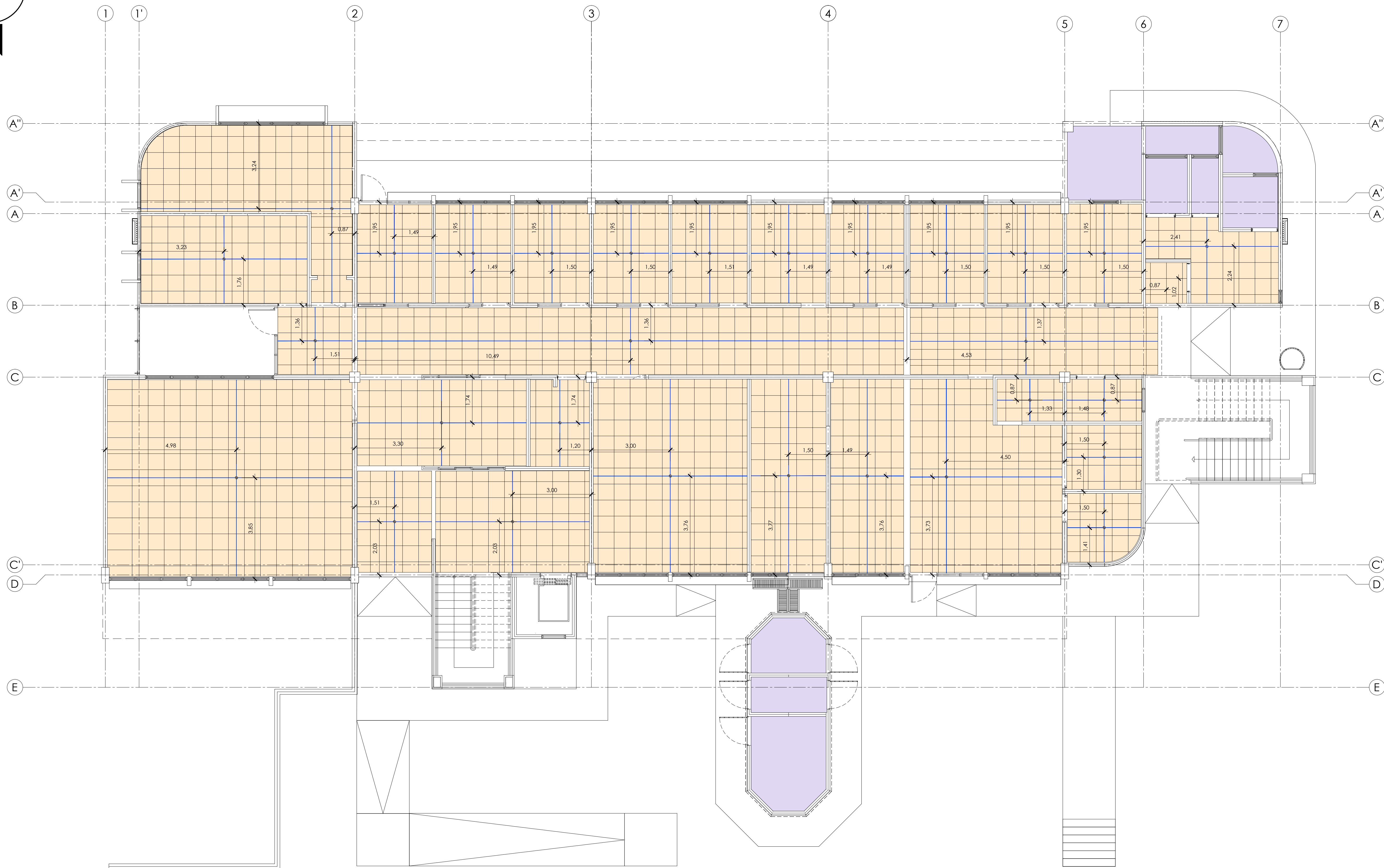
PLANTA ARQUITECTÓNICA DE CIELOS RASOS NIVEL 1
