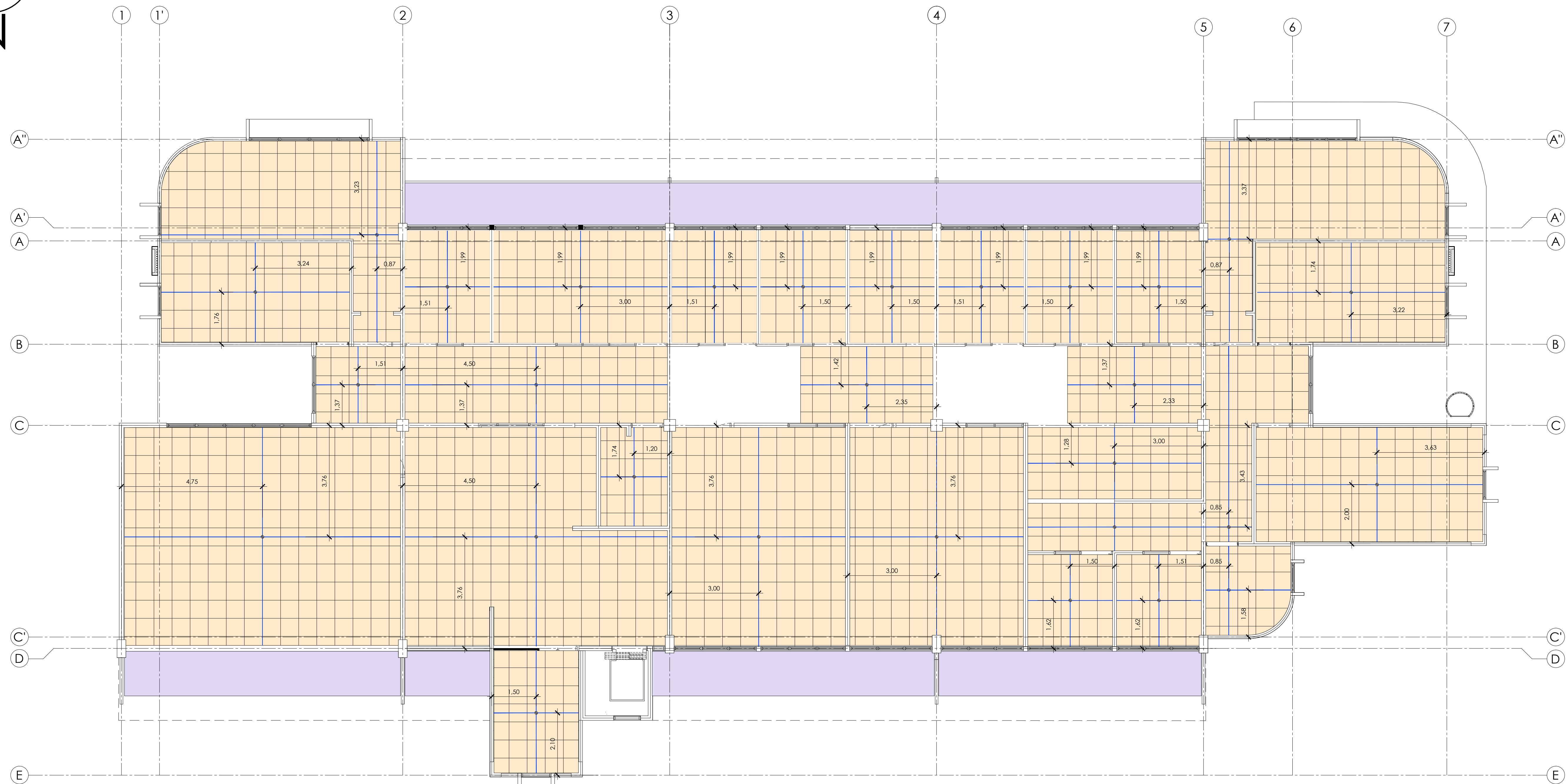
PLANTA ARQUITECTÓNICA DE CIELOS RASOS NIVEL 2 ESCALA 1:75
