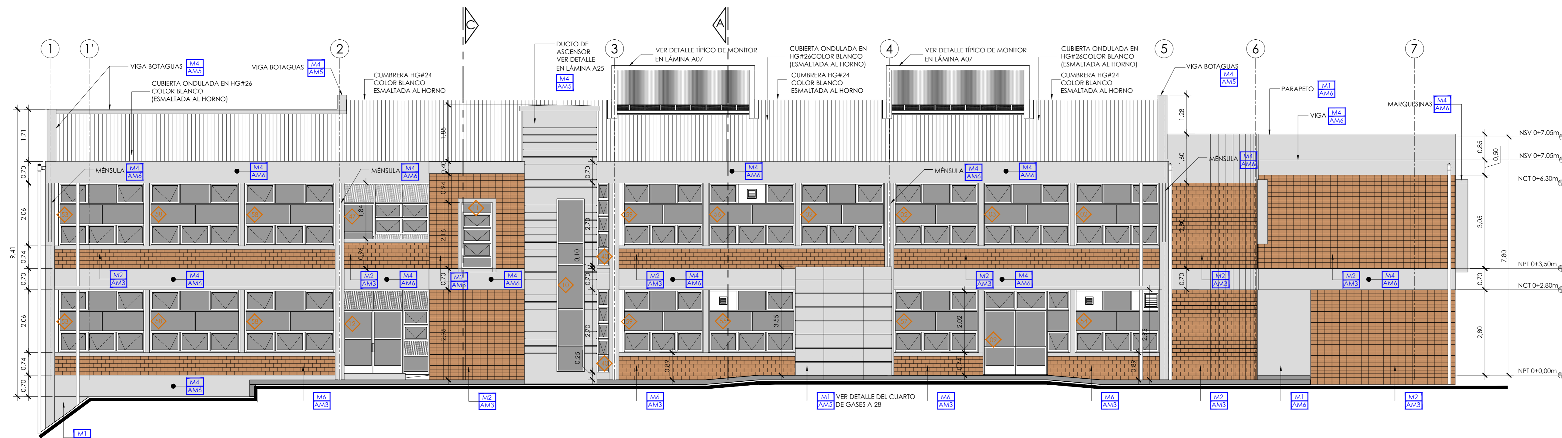
FACHADA NORTE PRINCIPAL CON CUARTO DE GASES ESCALA 1:75
