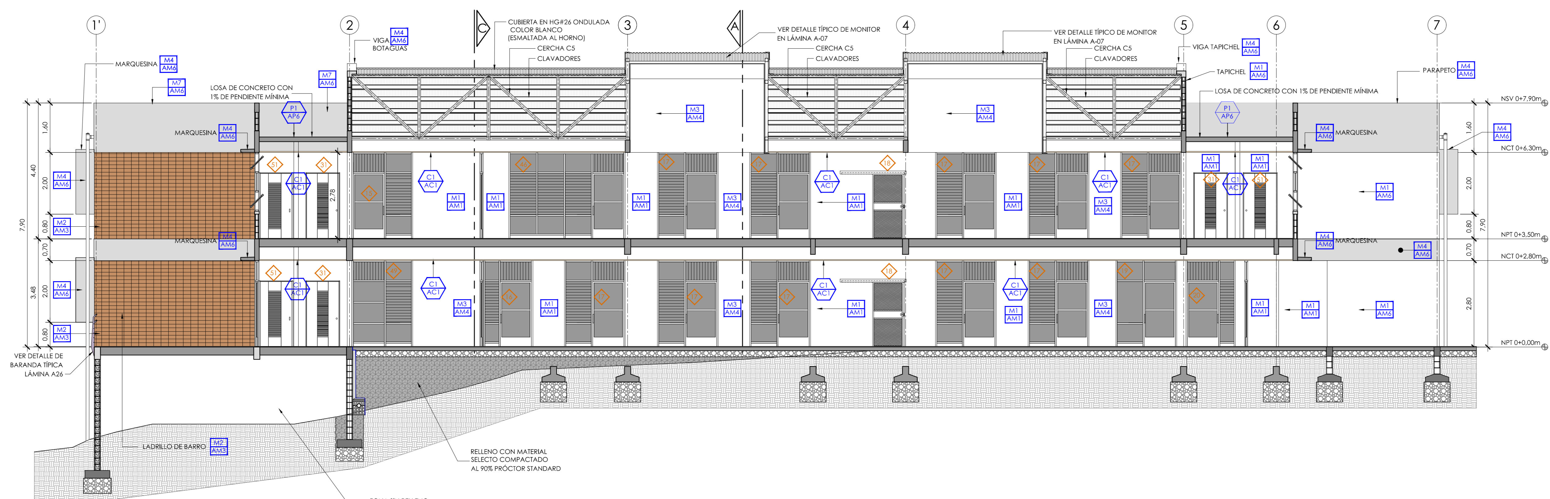
CORTE BB ESCALA 1:75
