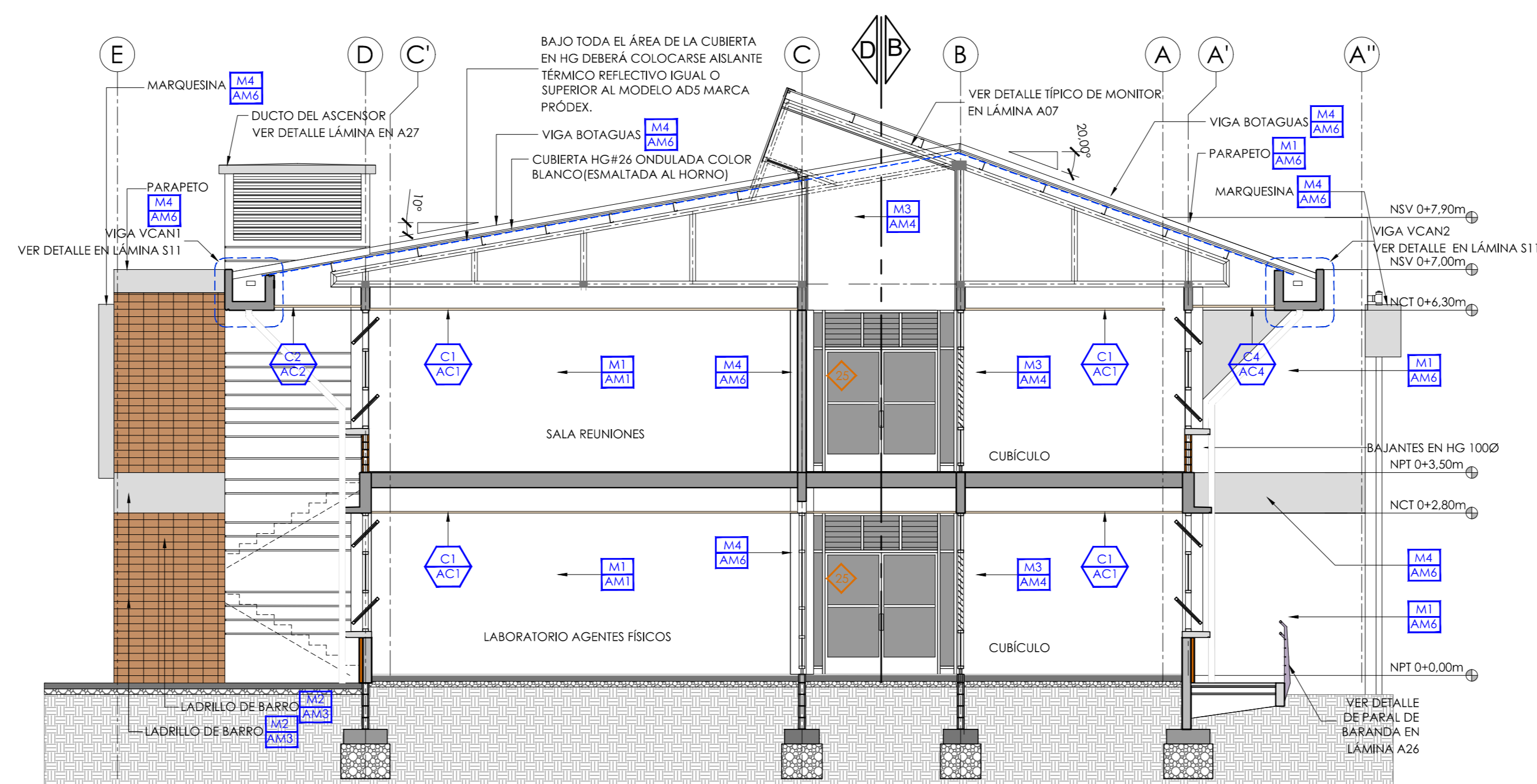
CORTE AA ESC. 1:75
