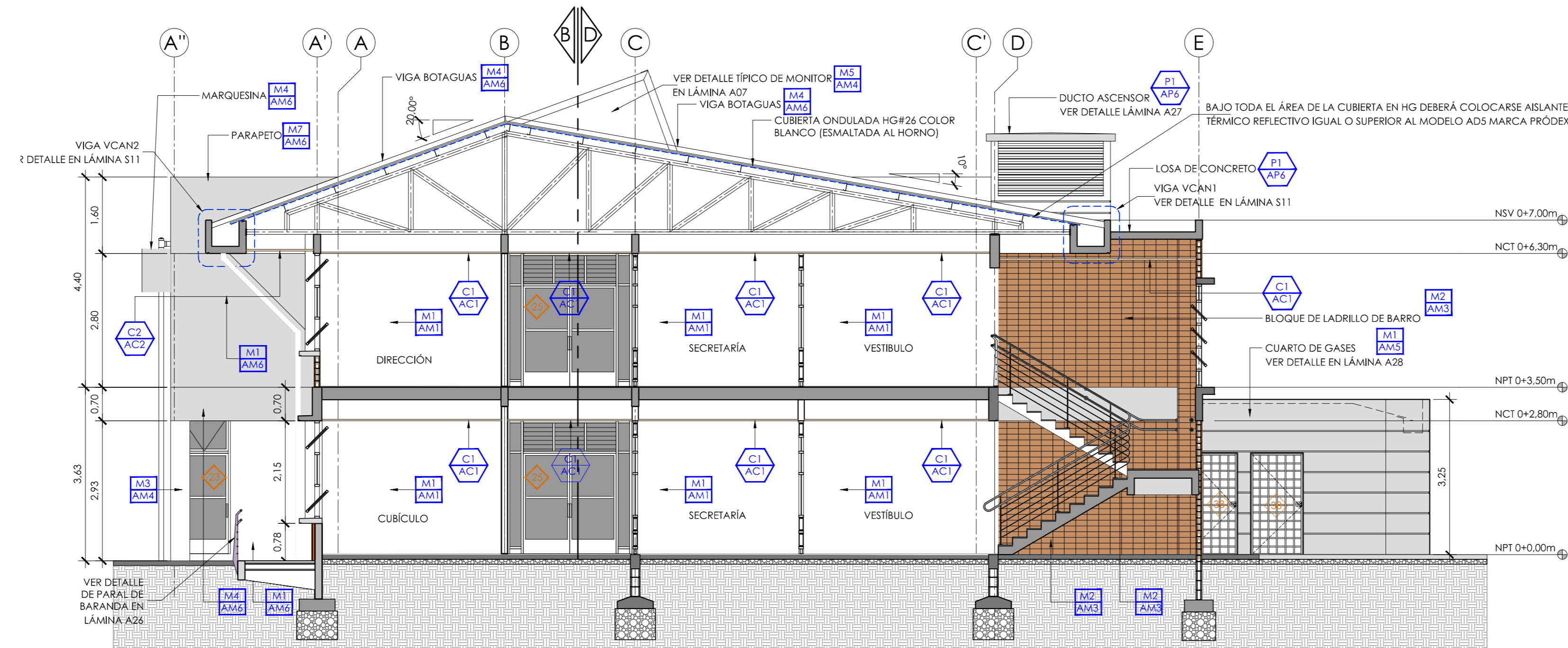
CORTE CC ESCALA 1:75
