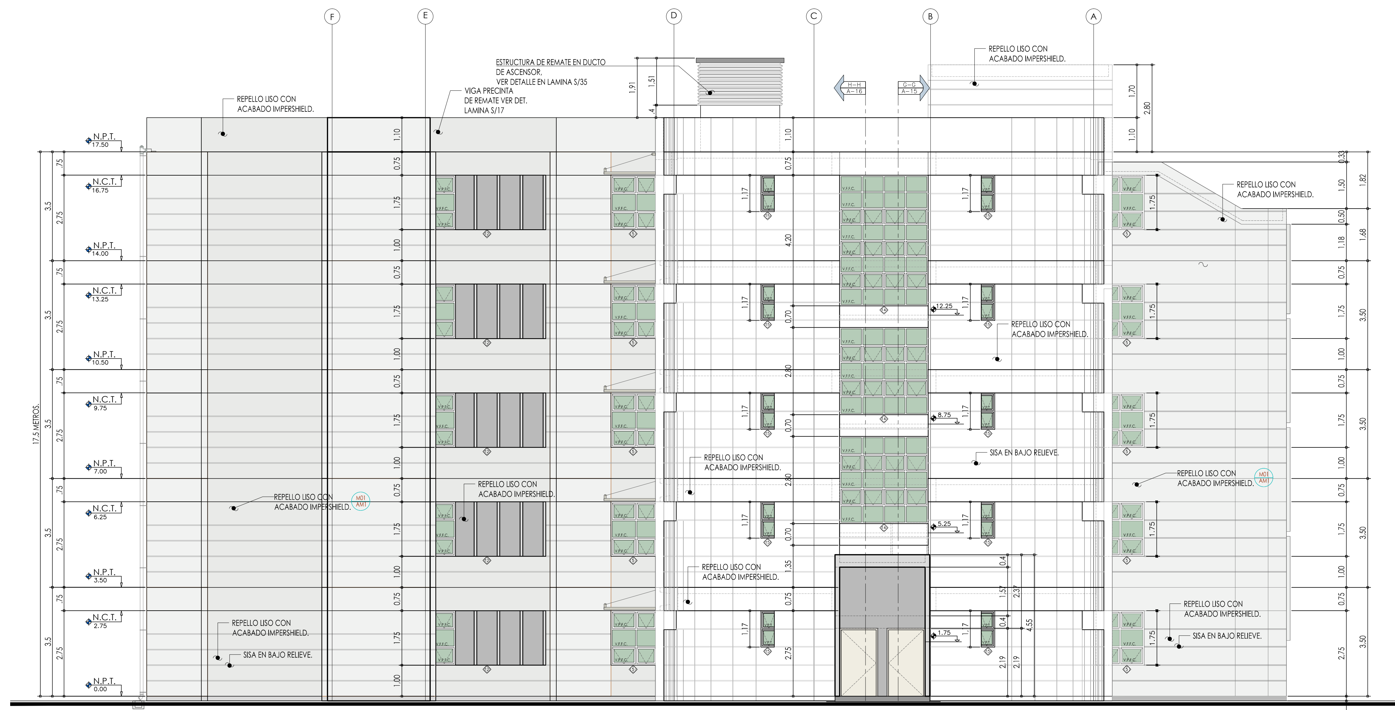
ELEVACION ESTE. ESCALA 1:75
