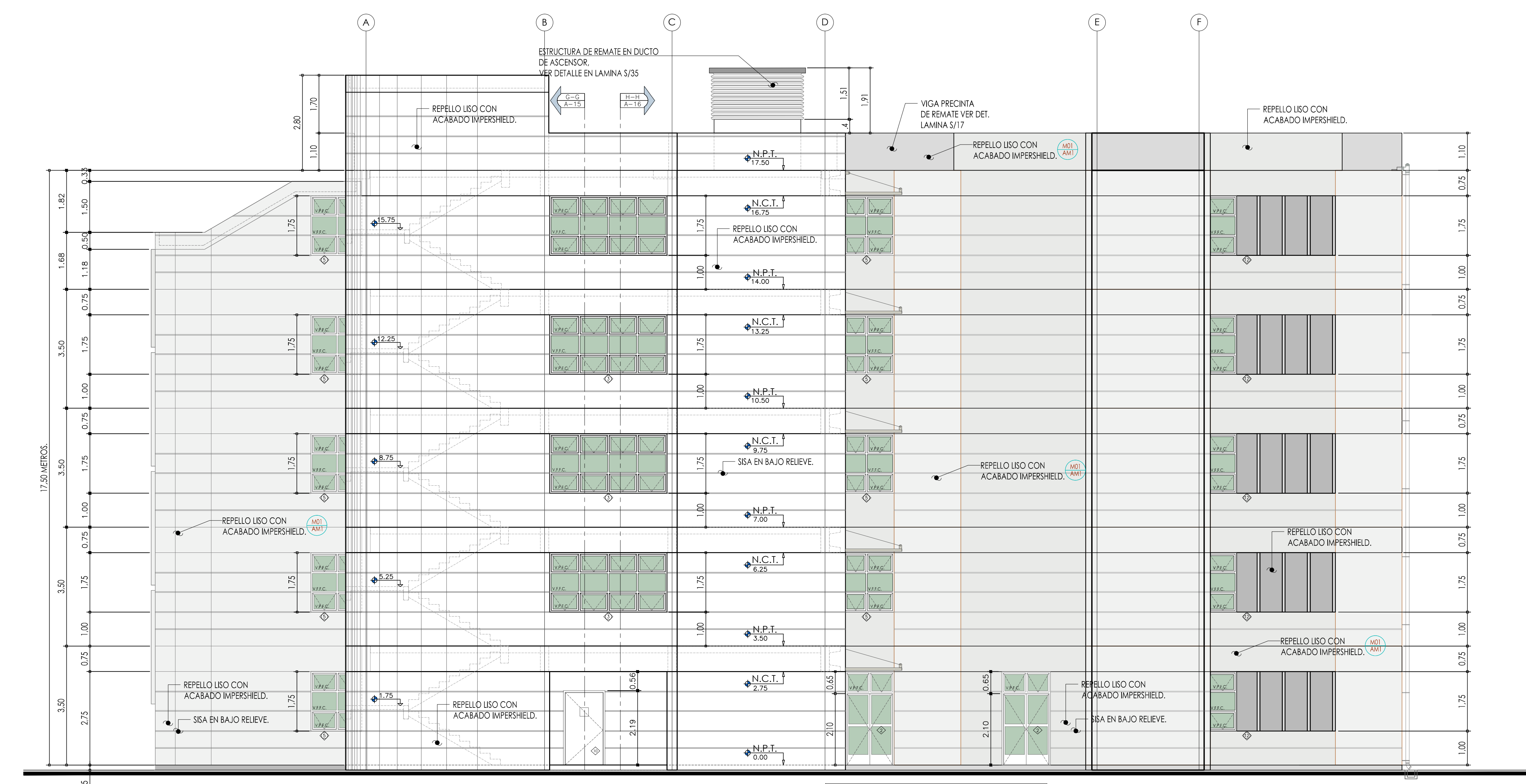
ELEVACION OESTE ESCALA 1:75
