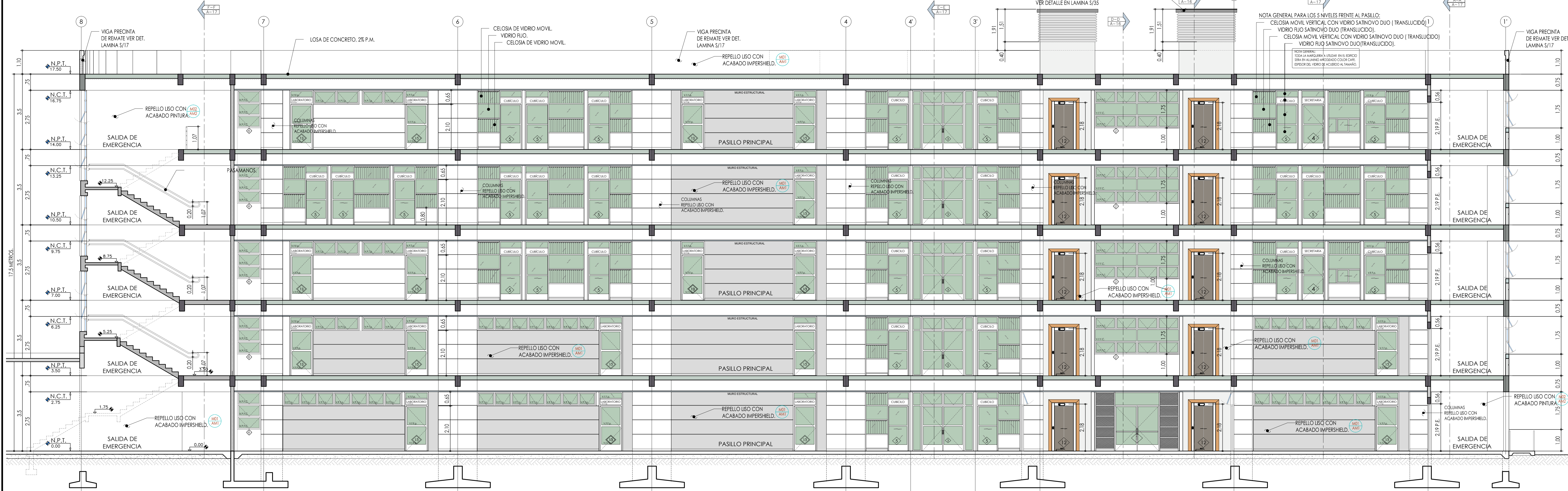
SECCIÓN HH ESCALA 1:75
