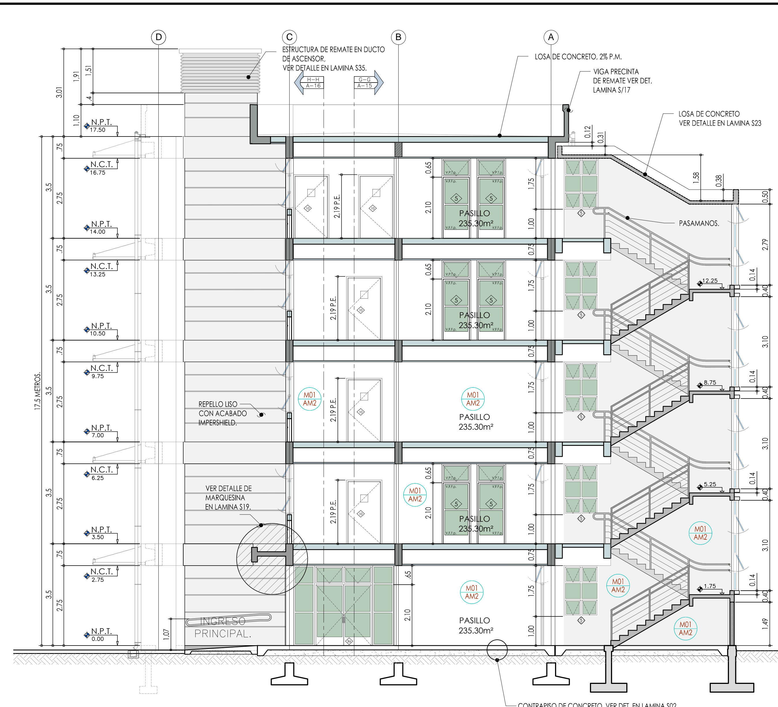
SECCIÓN DD ESCALA 1:75
