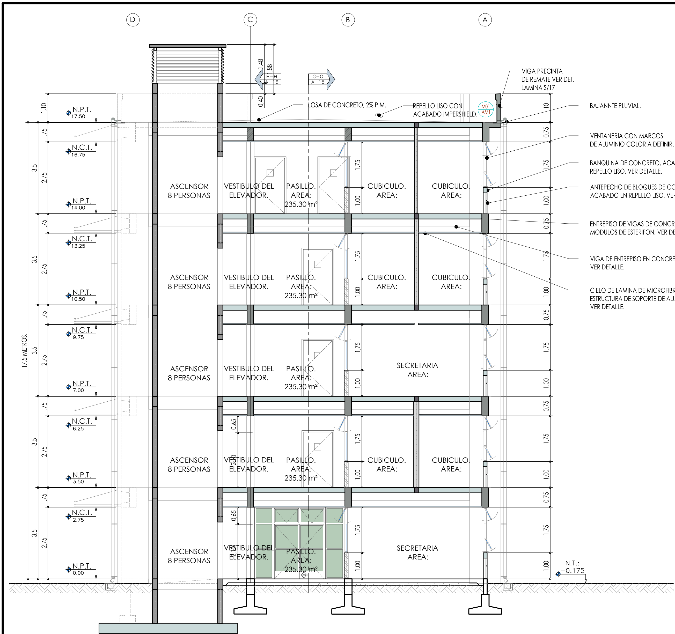
SECCIÓN CC ESCALA 1:75
