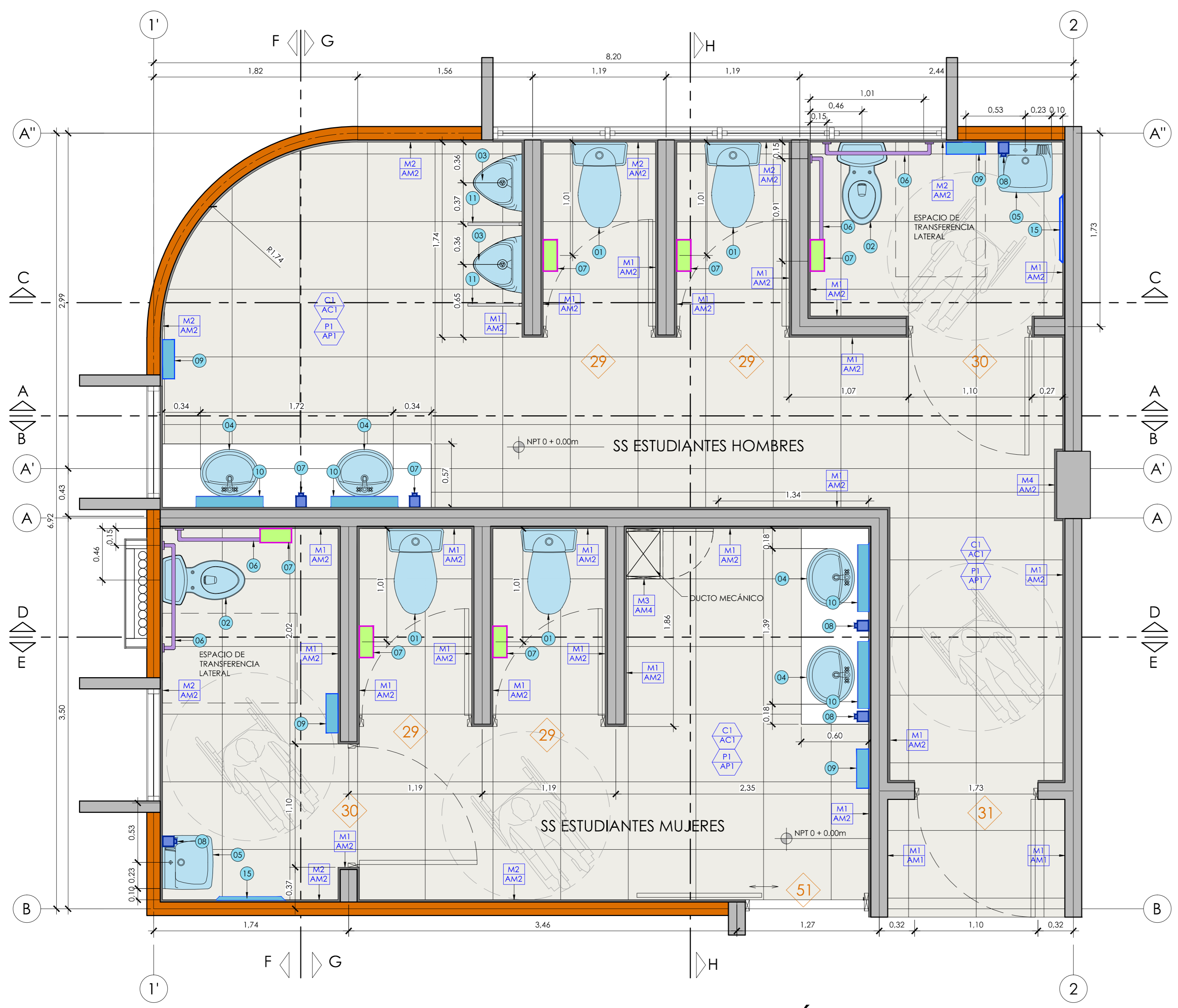
DETALLE AMPLIADO DE LA PLANTA DE BATERÍA SANITARIA TIPO 1 ESCALA 1:25
