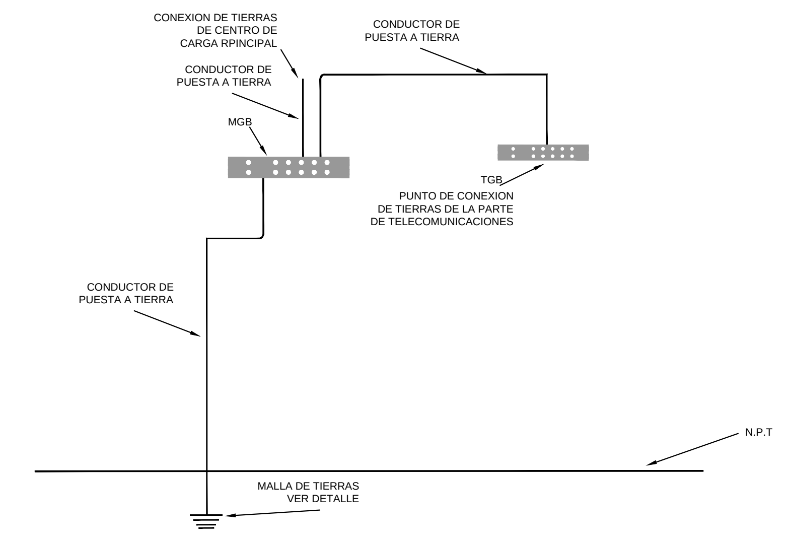
DETALLE DE SISTEMA MODULAR DE PUESTA A TIERRA PARA TELECOMUNICACIONES. SIN ESCALA.
