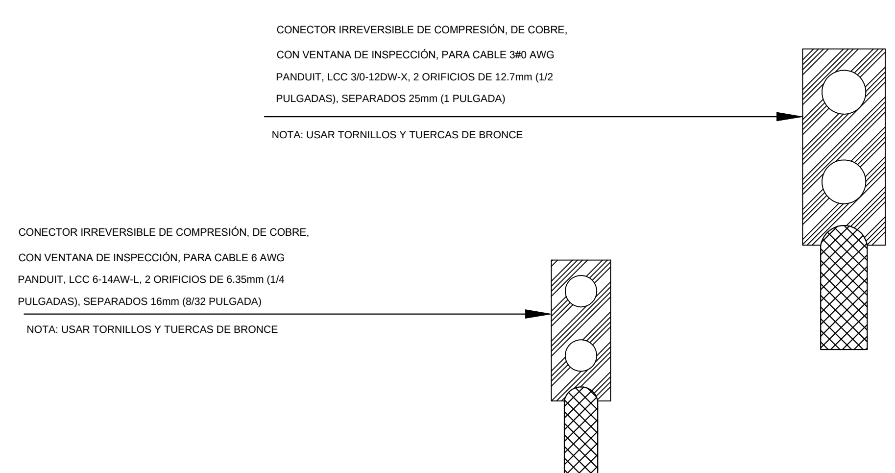
DETALLE DE CONECTORES PARA TMGB Y TGB SIN ESCALA
