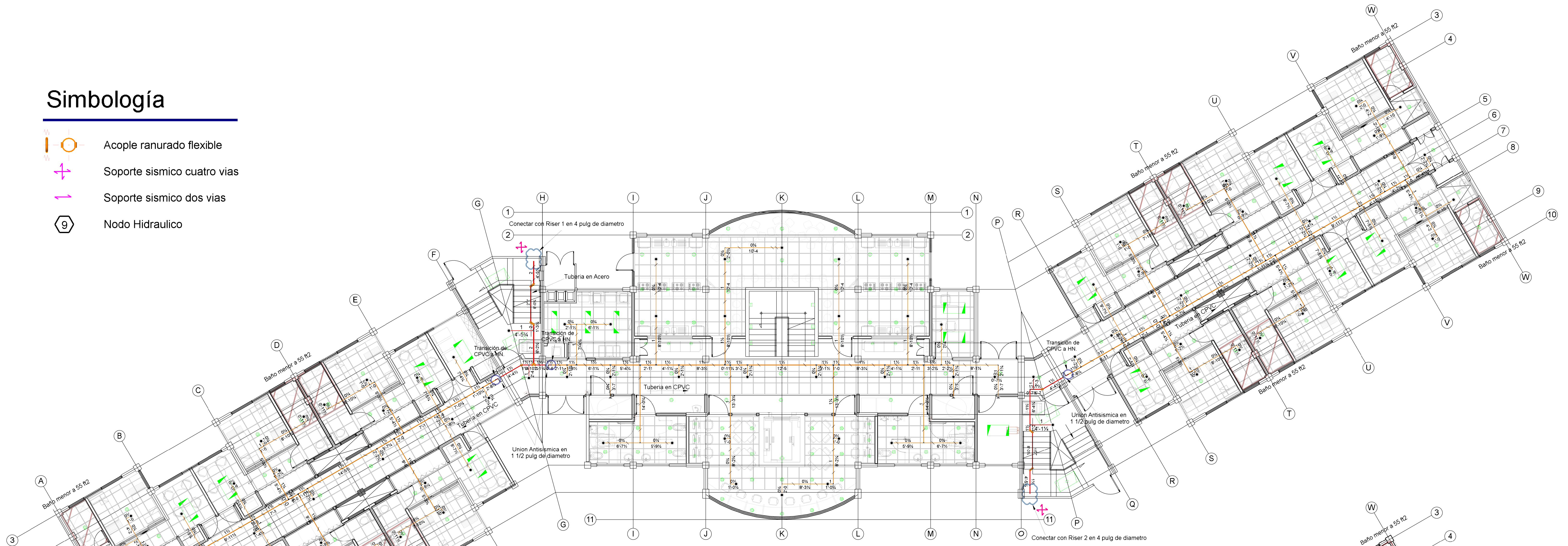
DISTRIBUCION PRINCIPAL PRIMER NIVEL SISTEMA DE PROTECCION CONTRA INCENDIOS ESCALA 1 = 100
