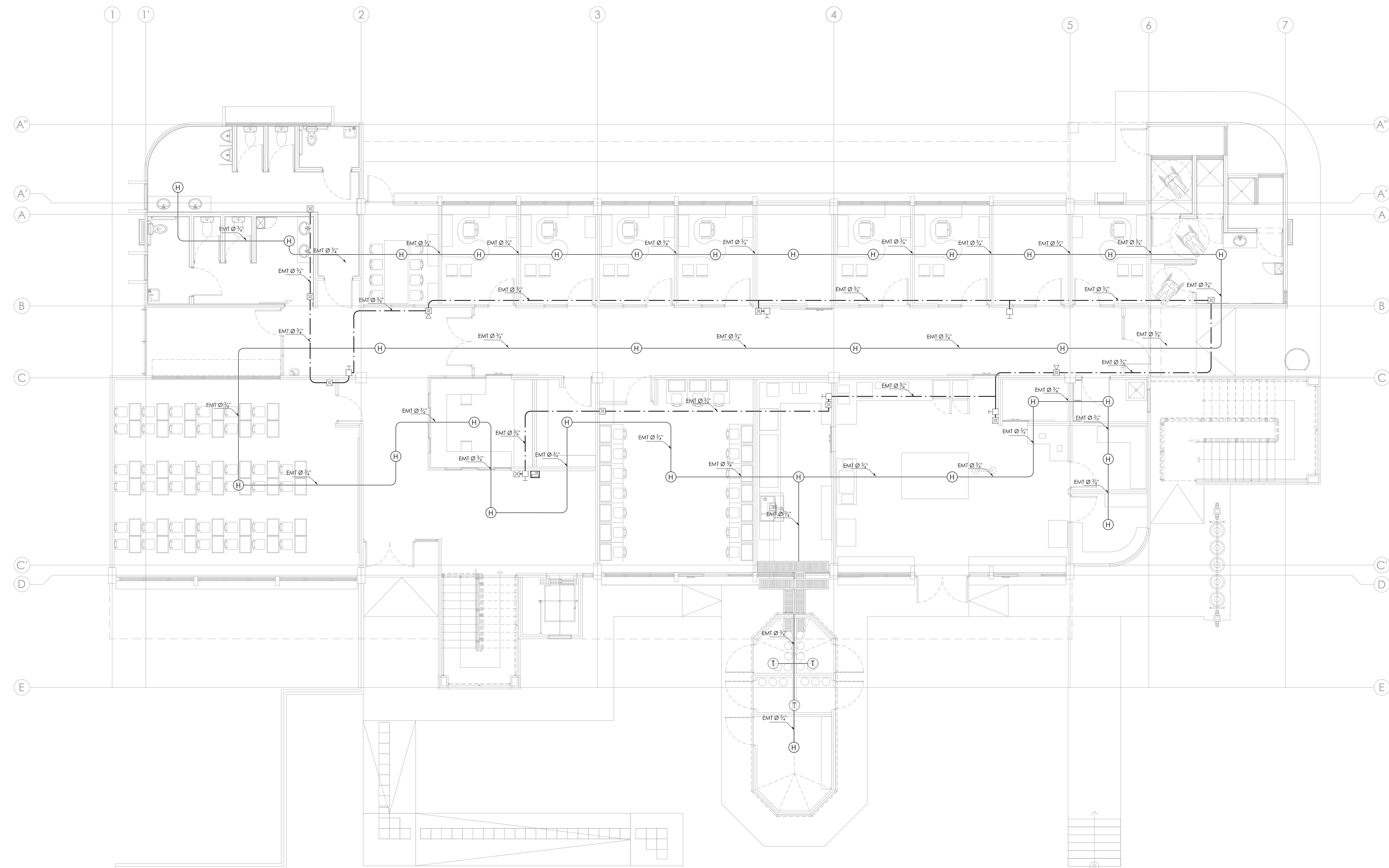
PLANTA DE SISTEMA DE DETECCION DE INCENDIO NIVEL 1 ESCALA 1:75
