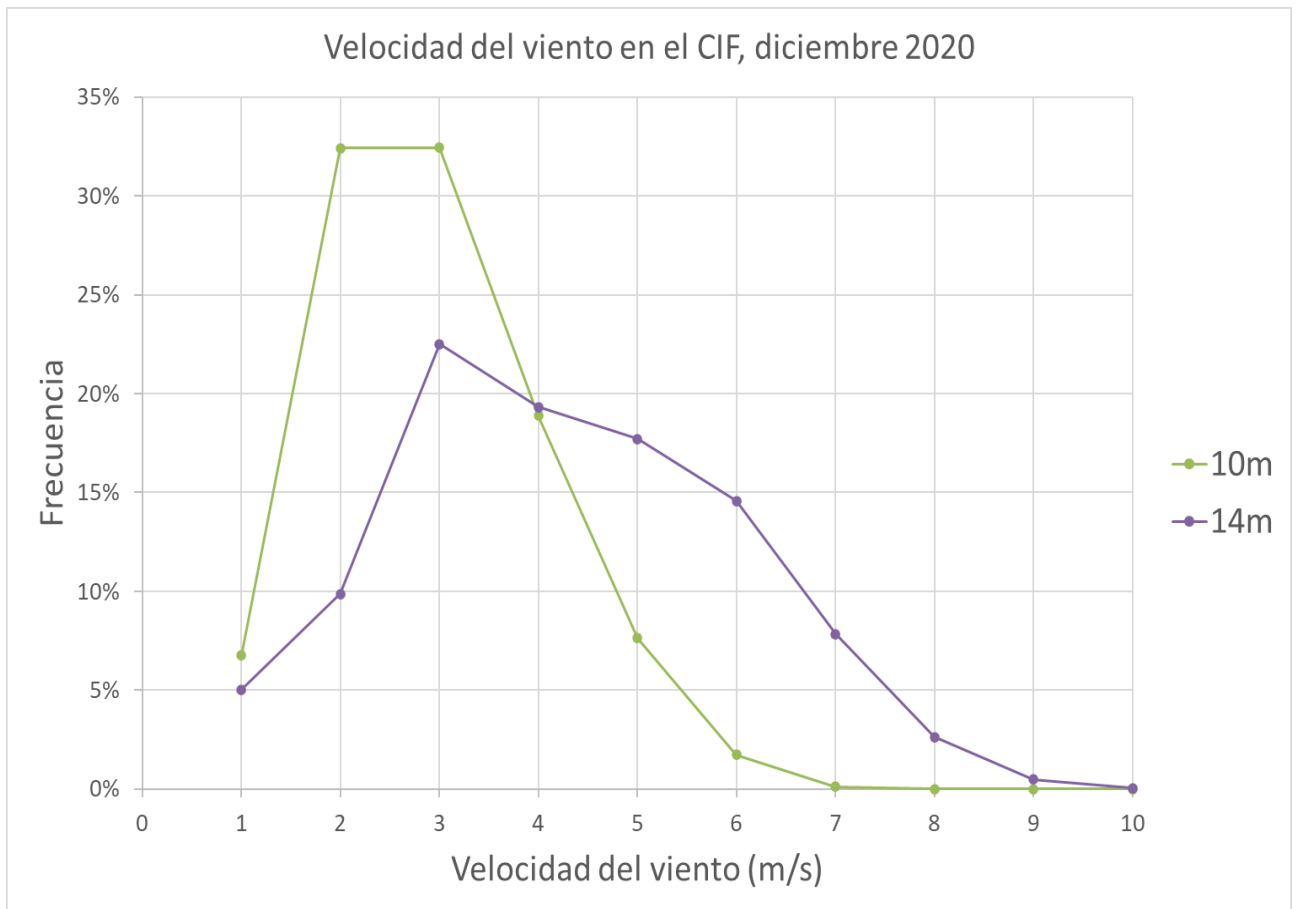
Figura 4. Velocidad del viento en la estación del CIF, diciembre 2020
