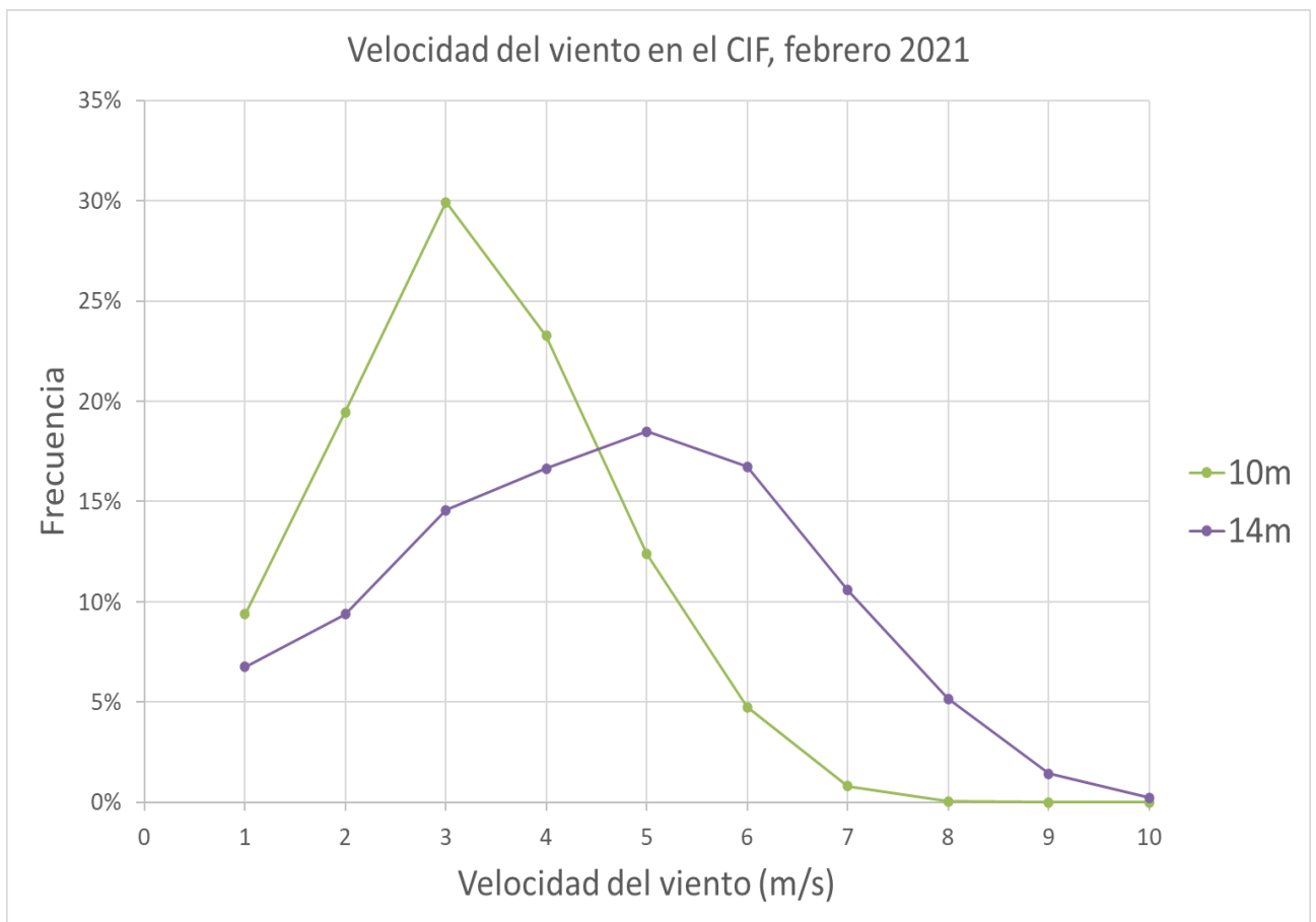
Figura 4. Velocidad del viento en la estación del CIF, febrero 2021
