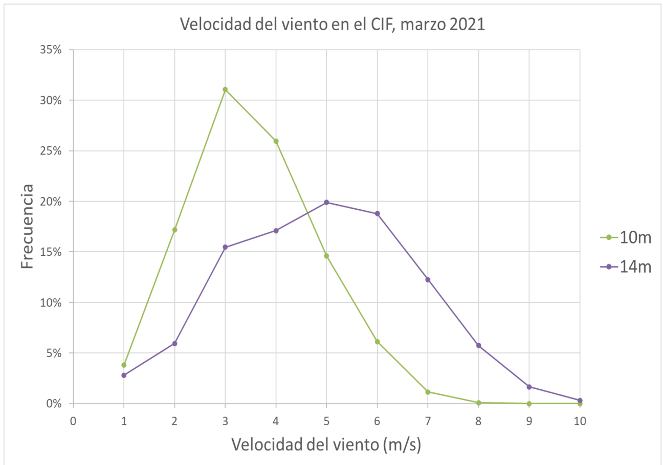
Figura 4. Velocidad del viento en la estación del CIF, marzo 2021
