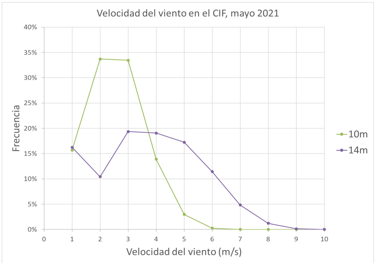
Figura 4. Velocidad del viento en la estación del CIF, mayo 2021
