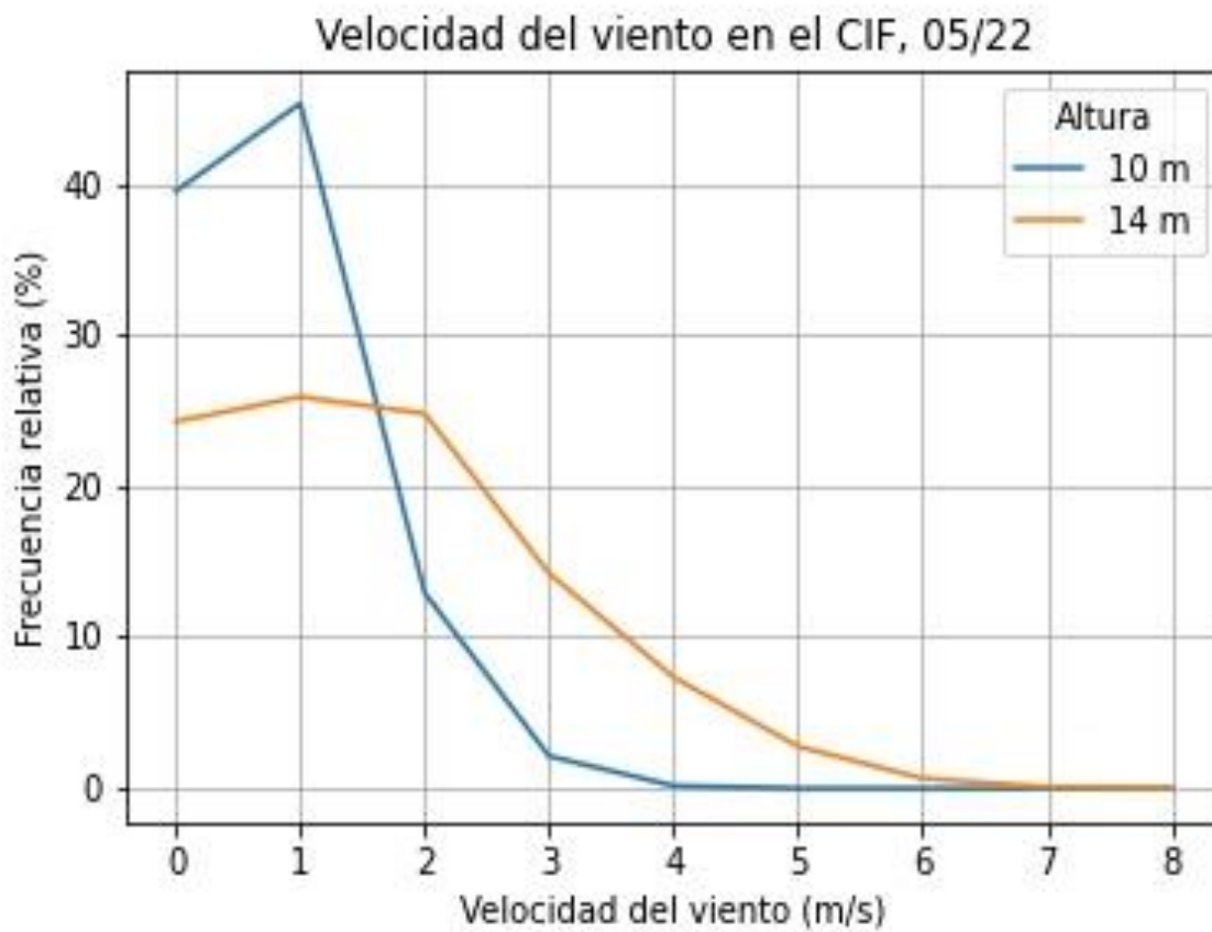
Figura 4. Histograma de la velocidad del viento en la estación del CIF, mayo 2022.
