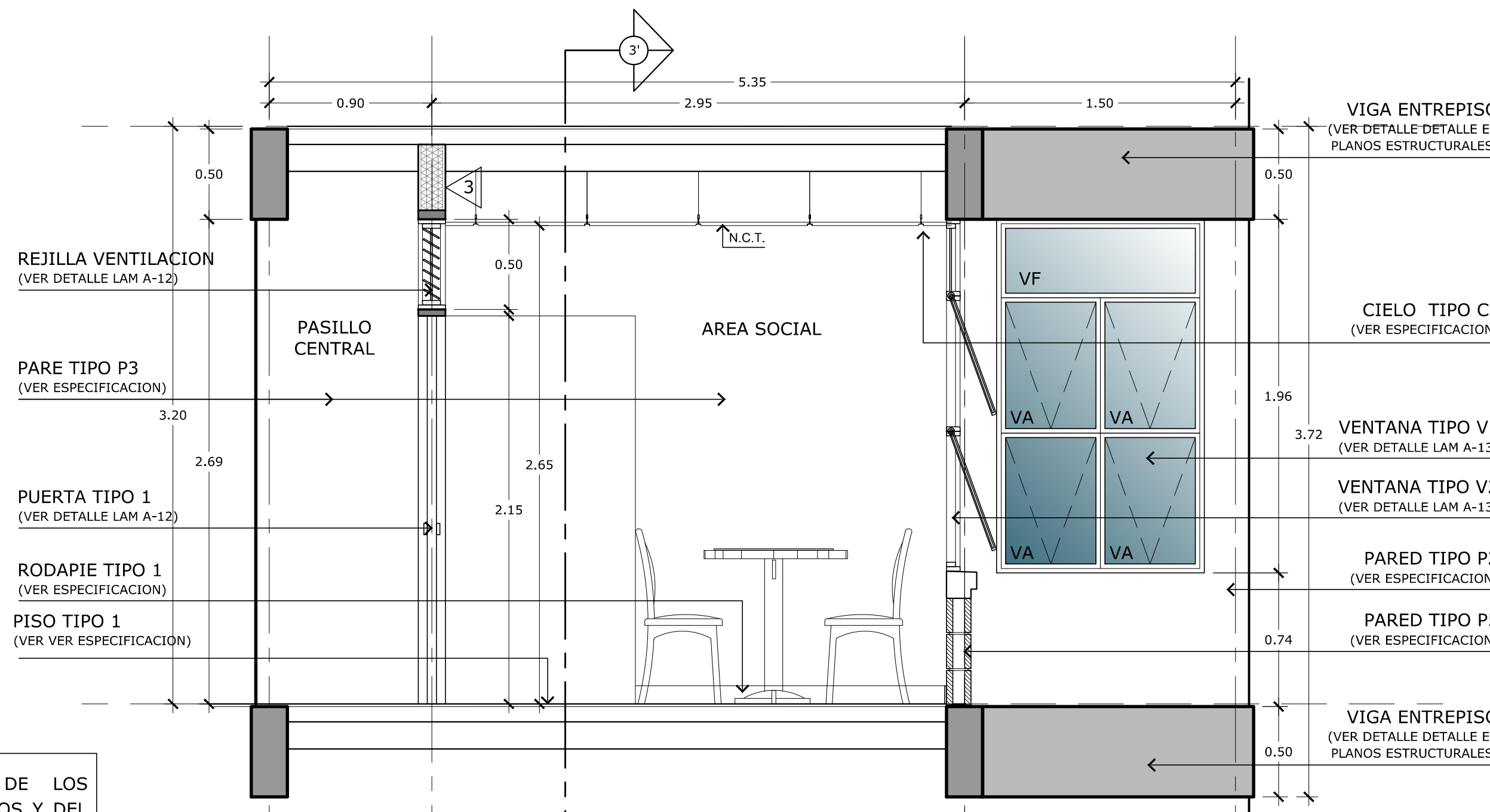
SECCION TRANSVERSAL 3-3 Esc: 1:25
