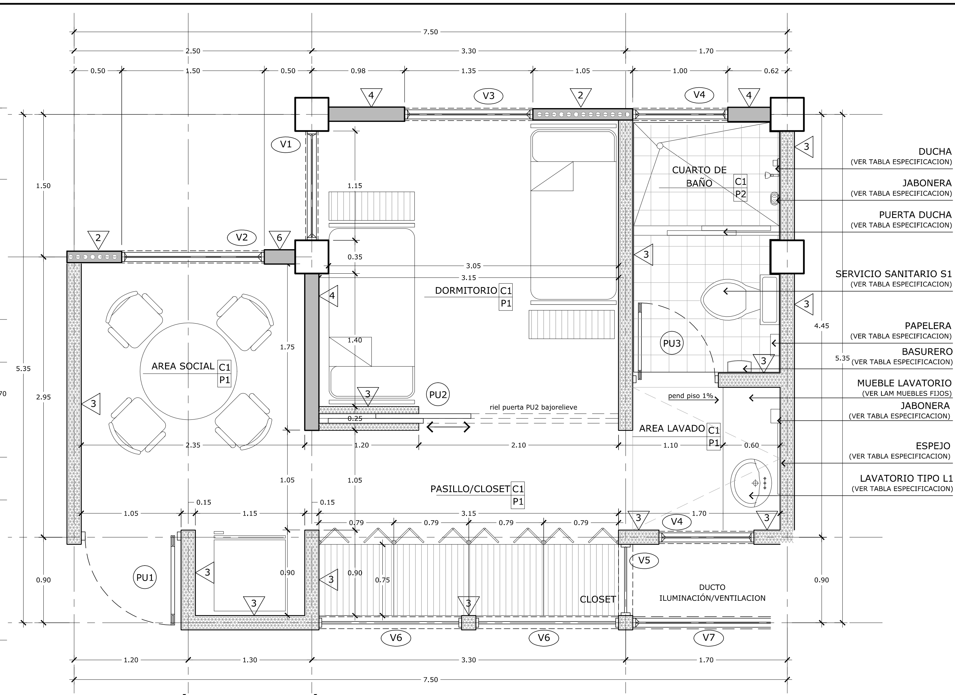
PLANTA DISTRIBUCIÓN ARQUITECTÓNICA. DORMITORIO TIPO 2 Esc: 1:25
