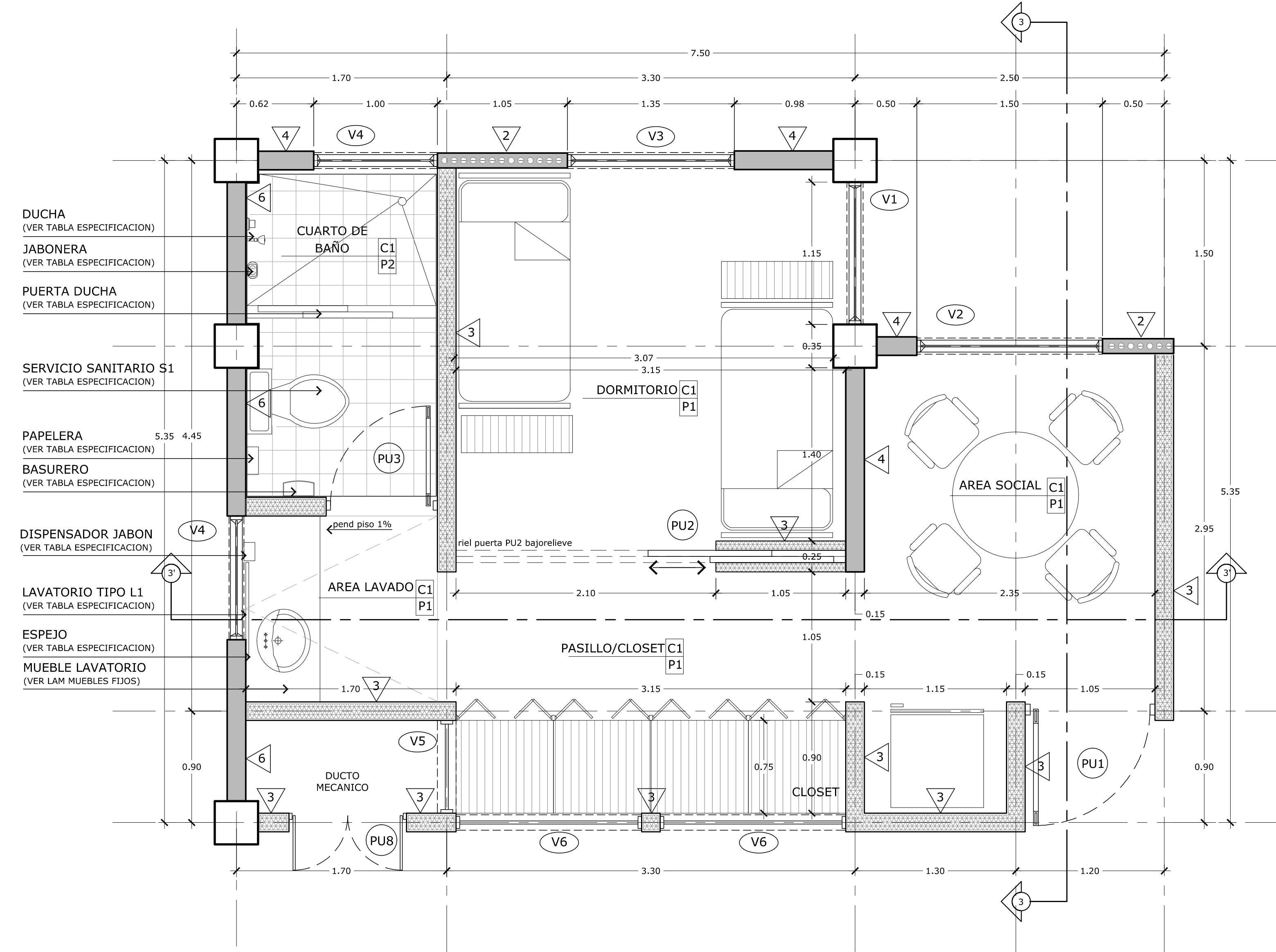
PLANTA DISTRIBUCIÓN ARQUITECTÓNICA. DORMITORIO TIPO 3 Esc: 1:25
