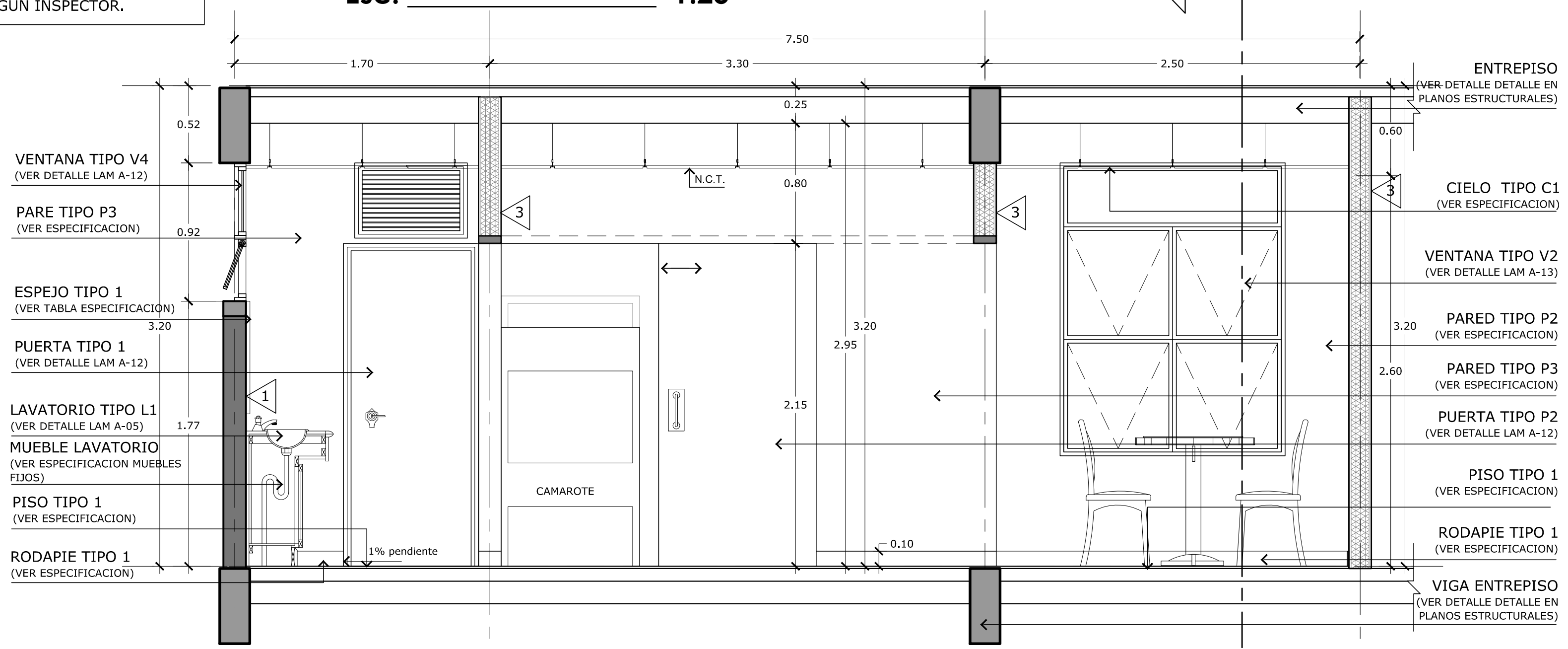
SECCION LONGITUDINAL 3'-3' Esc: 1:25
