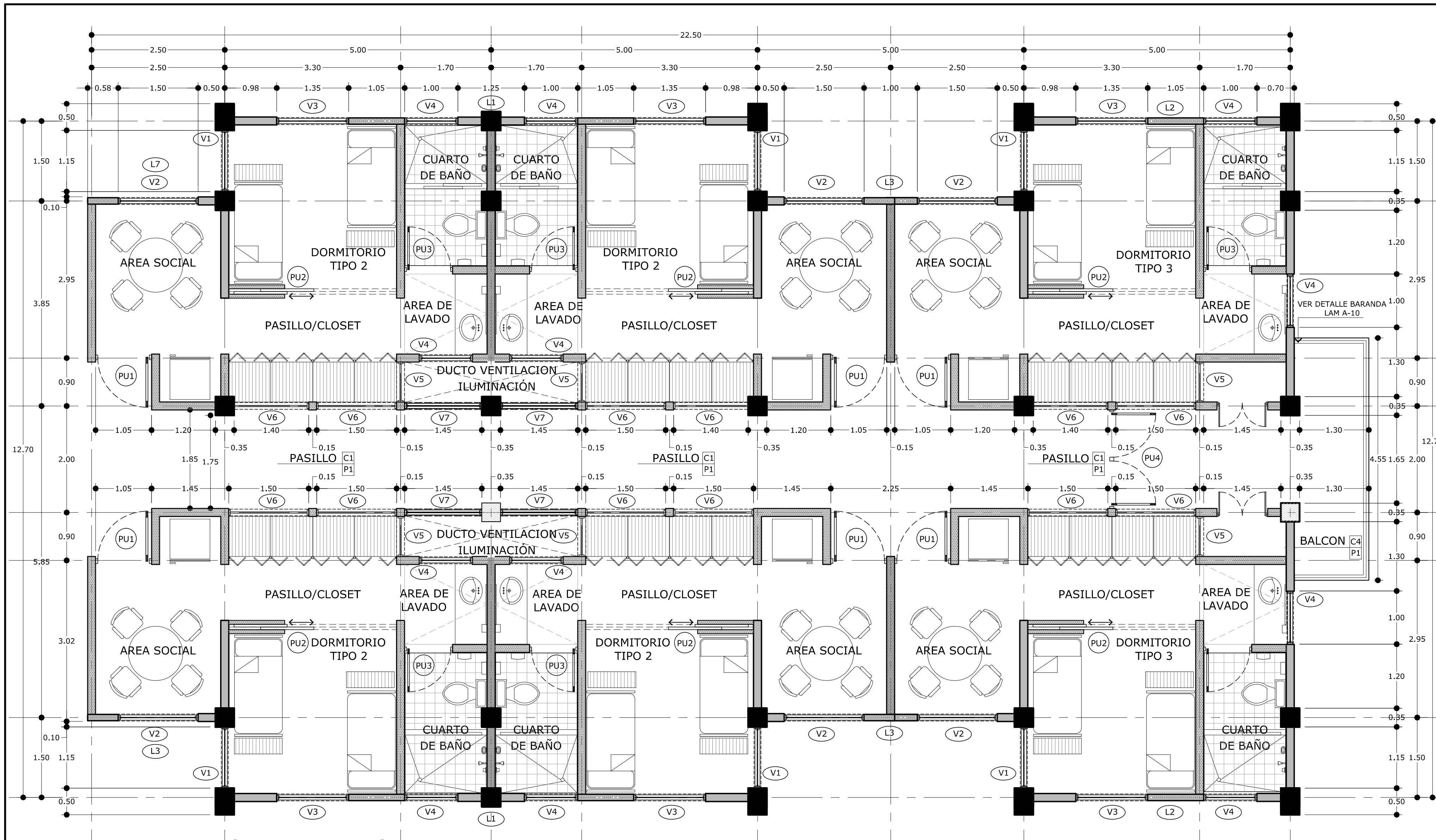
PLANTA DISTRIBUCIÓN ARQUITECTÓNICA ALA. TÍPICA DE DORMITORIOS NIVELES 3-4 Esc: 1:50
