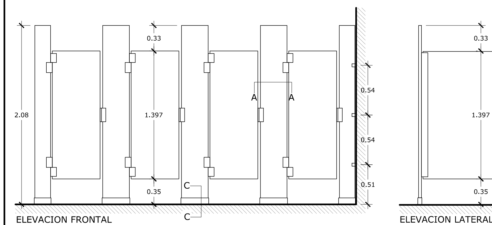
ELEVACION TÍPICO PARTICIONES METALICAS SS Esc: 1:25
