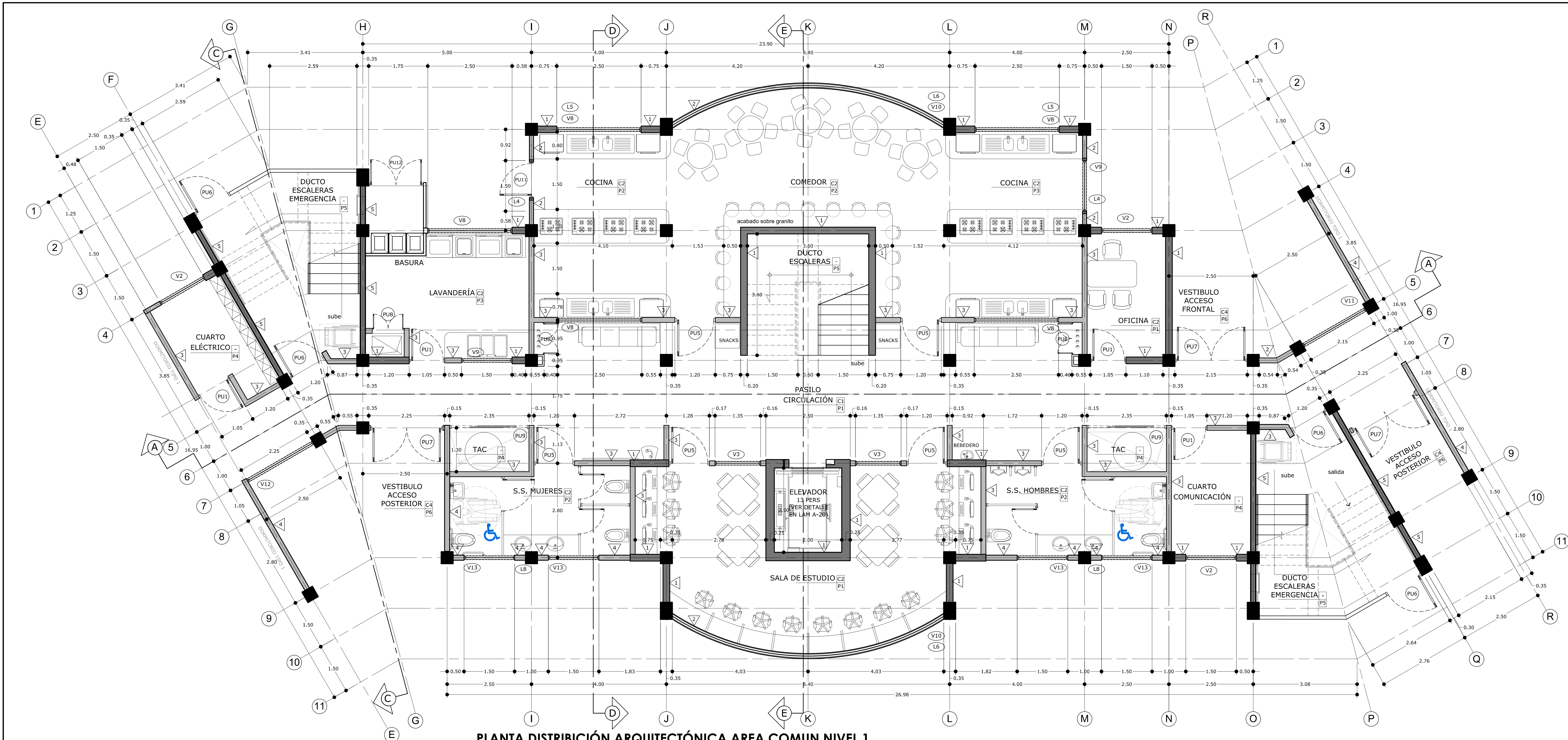
PLANTA DISTRIBUCIÓN ARQUITECTÓNICA AREA COMUN NIVEL 1 Esc: 1:50
