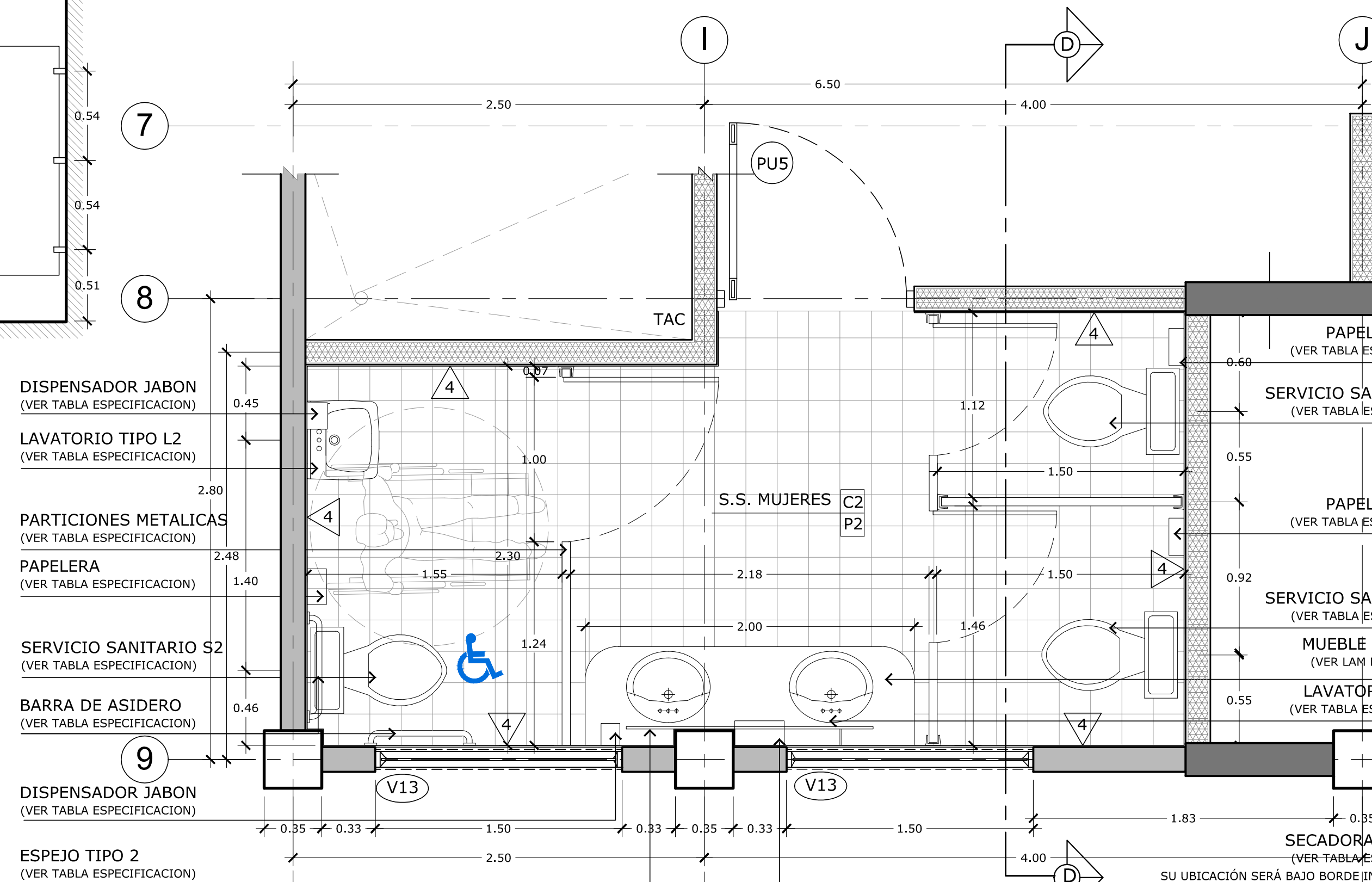
DETALLE TÍPICO BATERIA SERVICIOS SANITARIOS MUJERES Esc: 1:25
