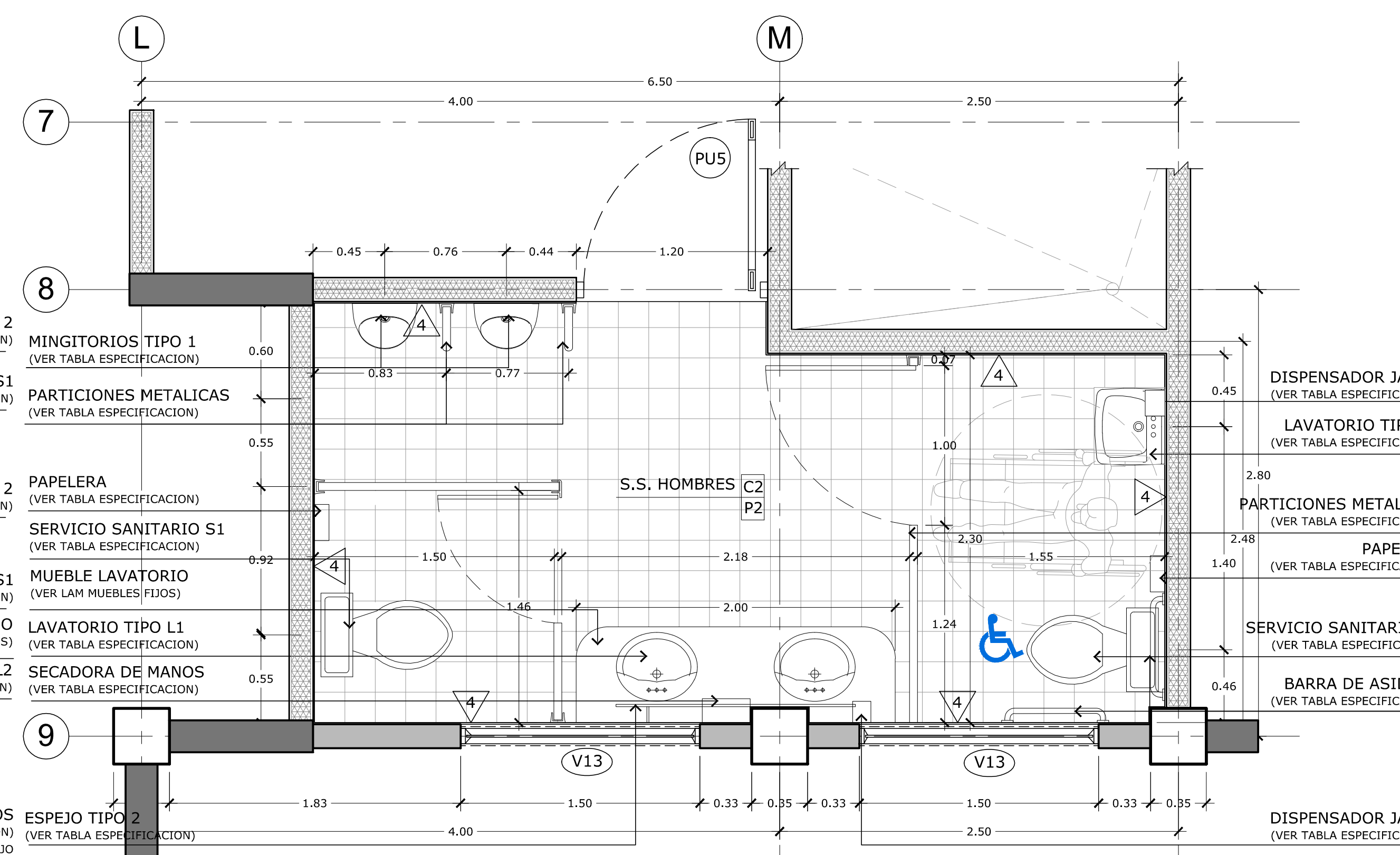
DETALLE TÍPICO BATERIA SERVICIOS SANITARIOS HOMBRES Esc: 1:25
