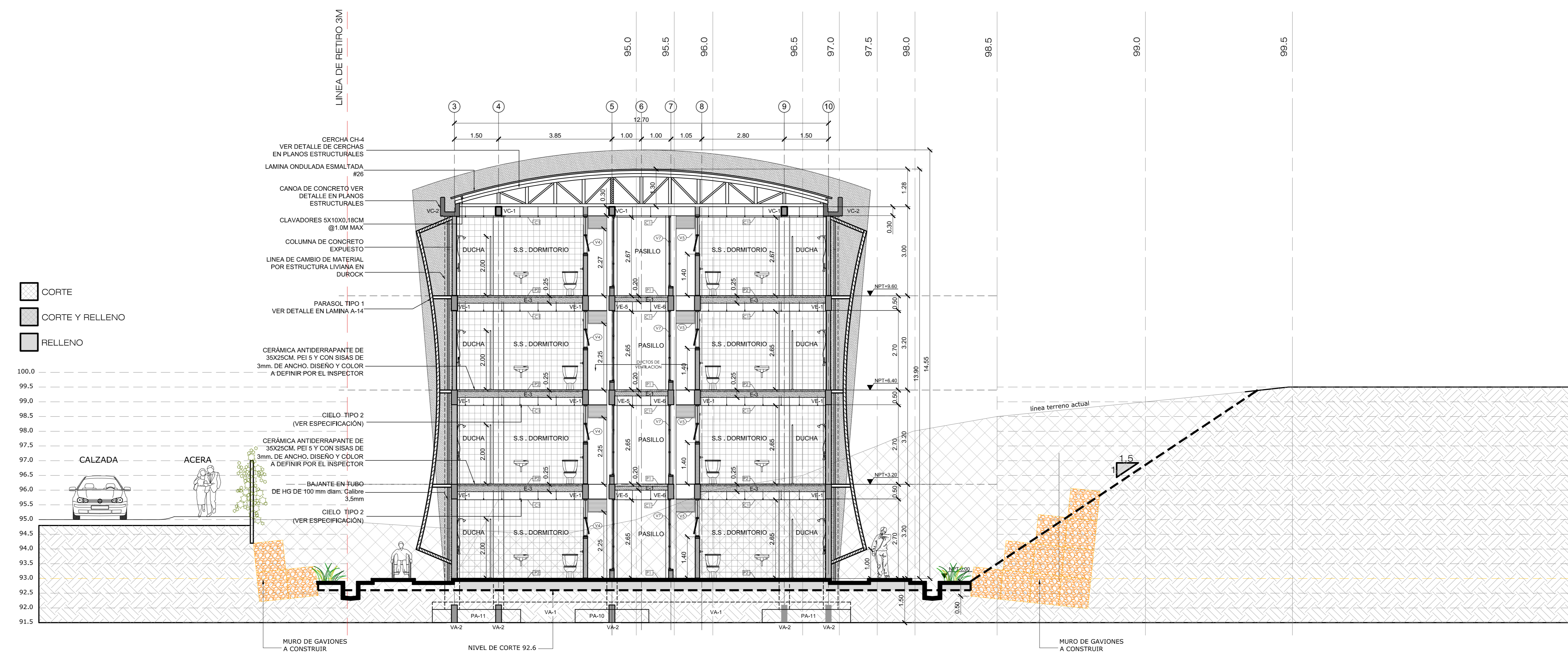
SECCION TRANSVERSAL B-B ESC 1:75
