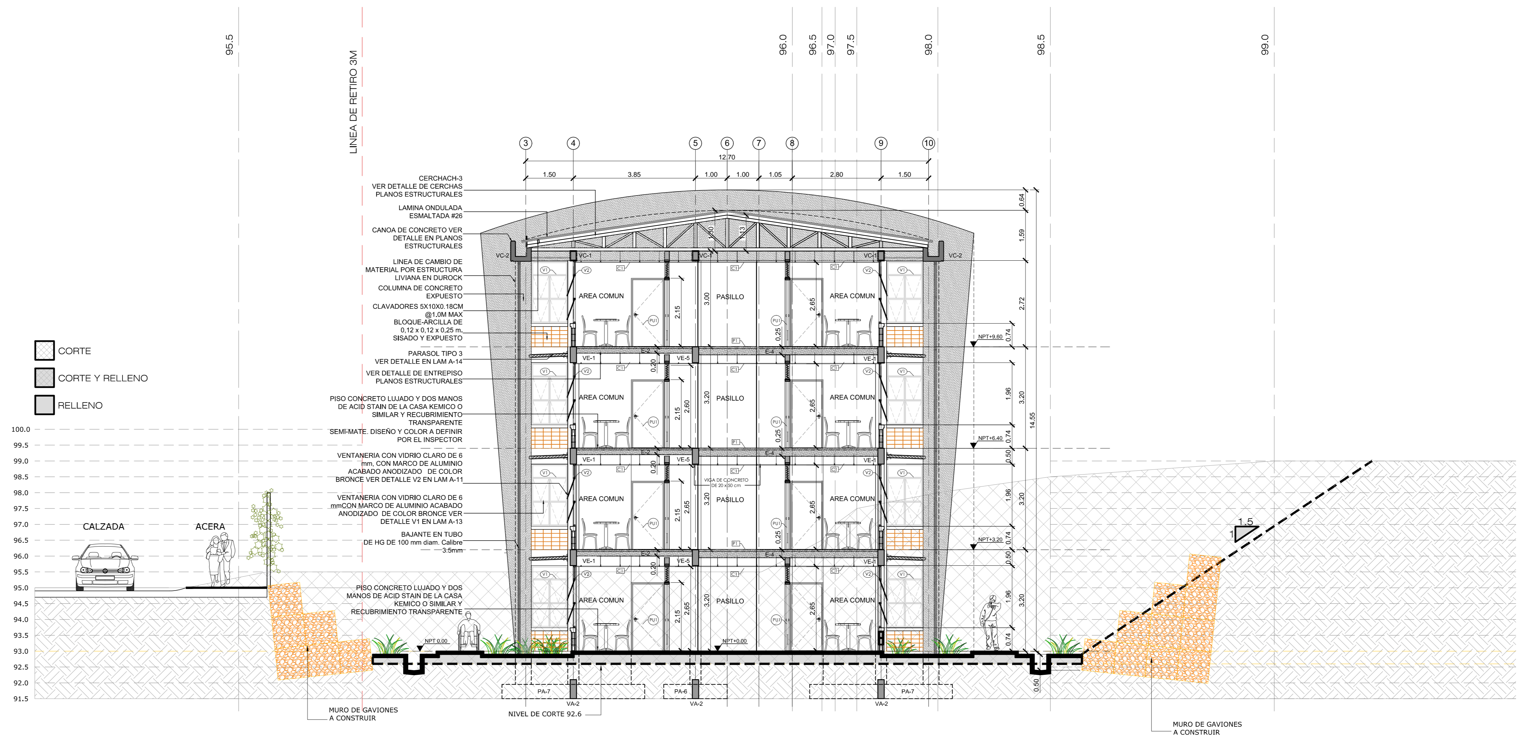
SECCION TRANSVERSAL A-A ESC 1:75
