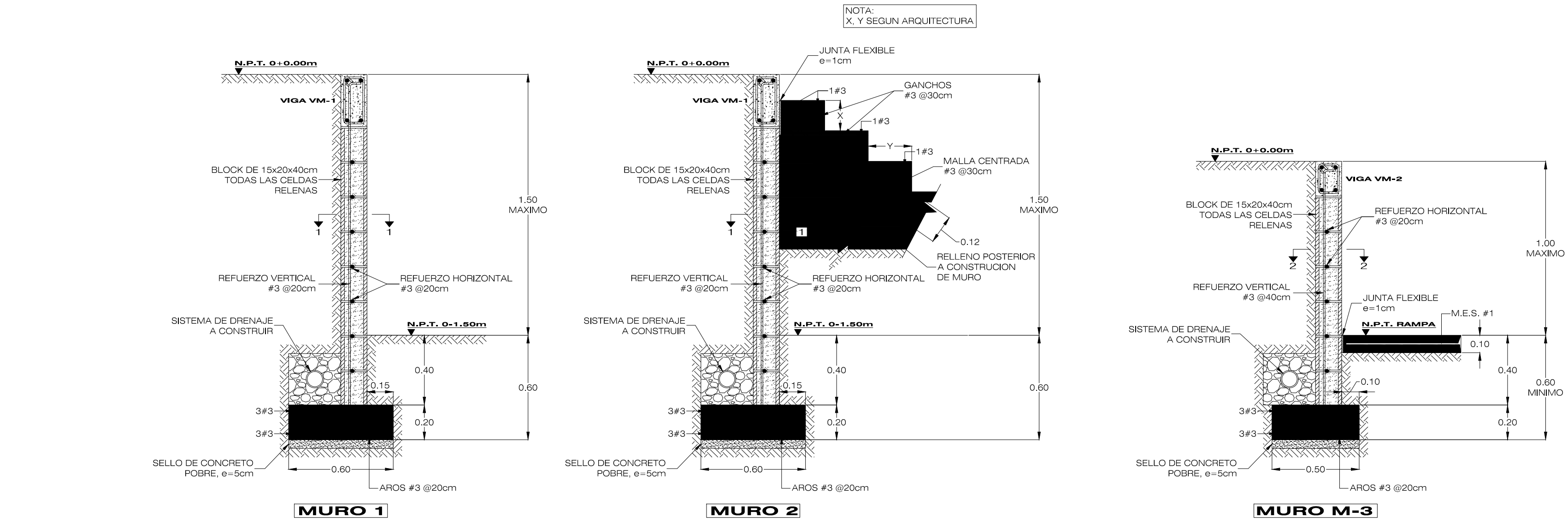
DETALLES DE MUROS ESCALA 1:20
