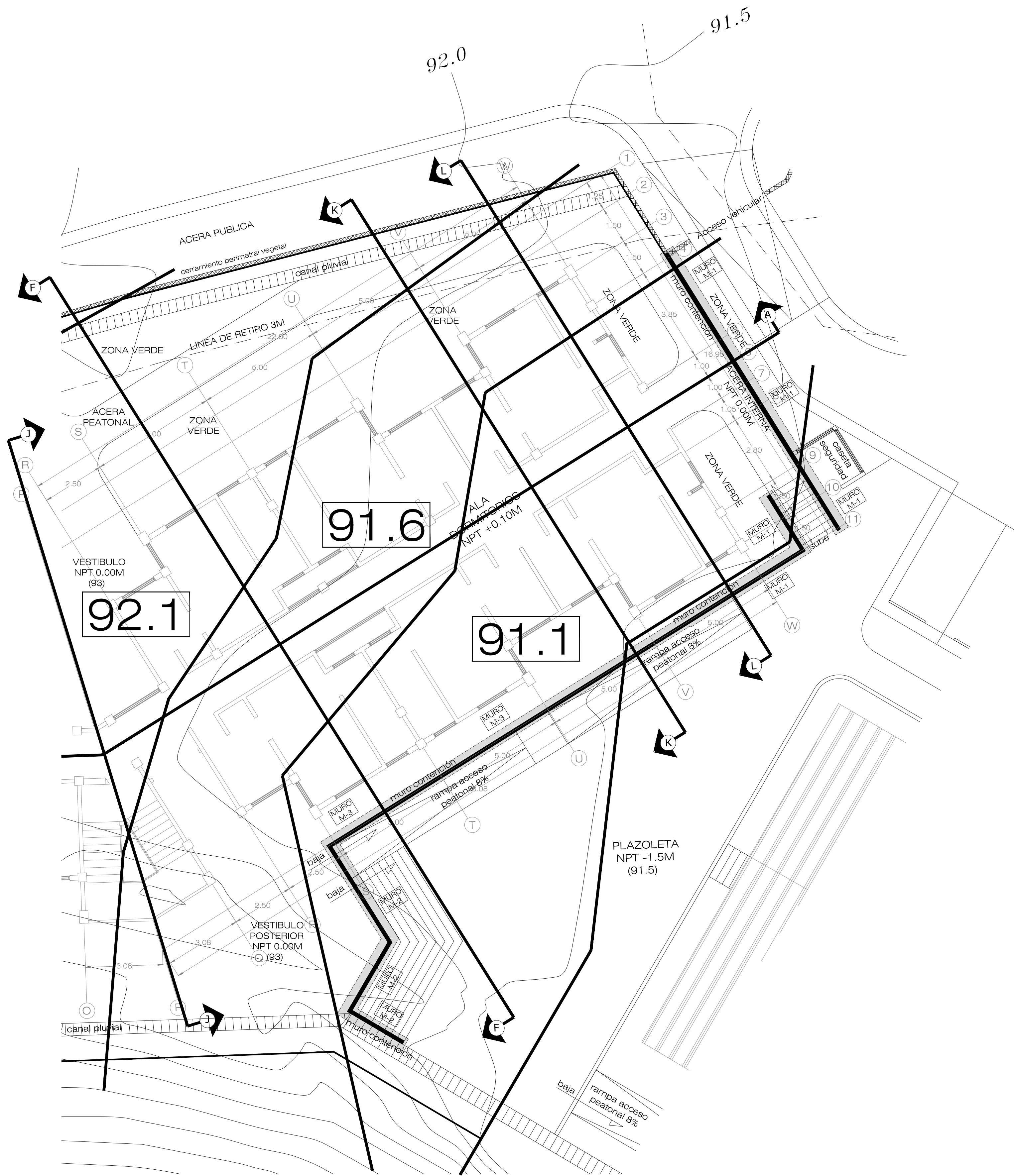
PLANTA DE MUROS ZONA 2 ESCALA 1:100
