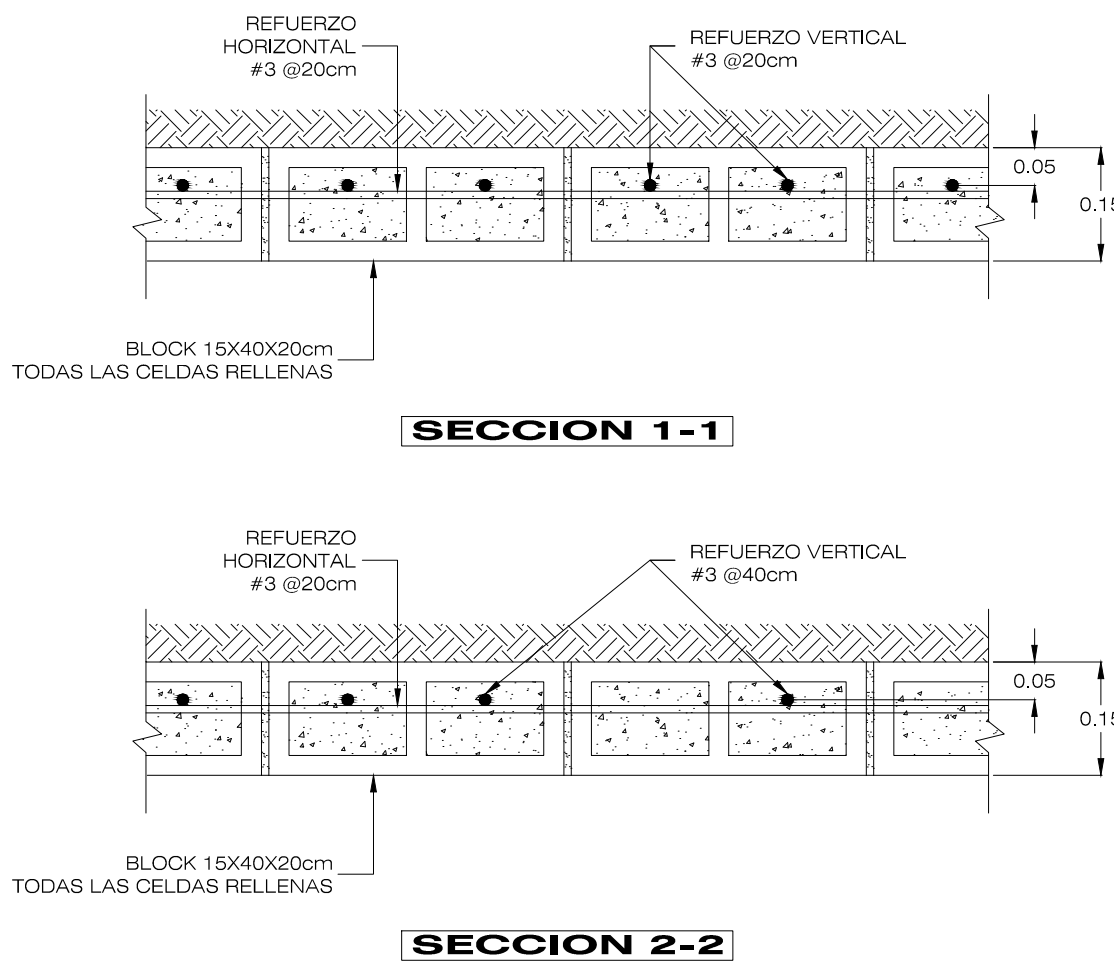
DETALLES SECCIONES DE MUROS ESCALA 1:10
