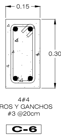
DETALLE COLUMNA DE MUROS ESCALA 1:10
