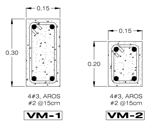
DETALLES VIGAS DE MUROS ESCALA 1:10
