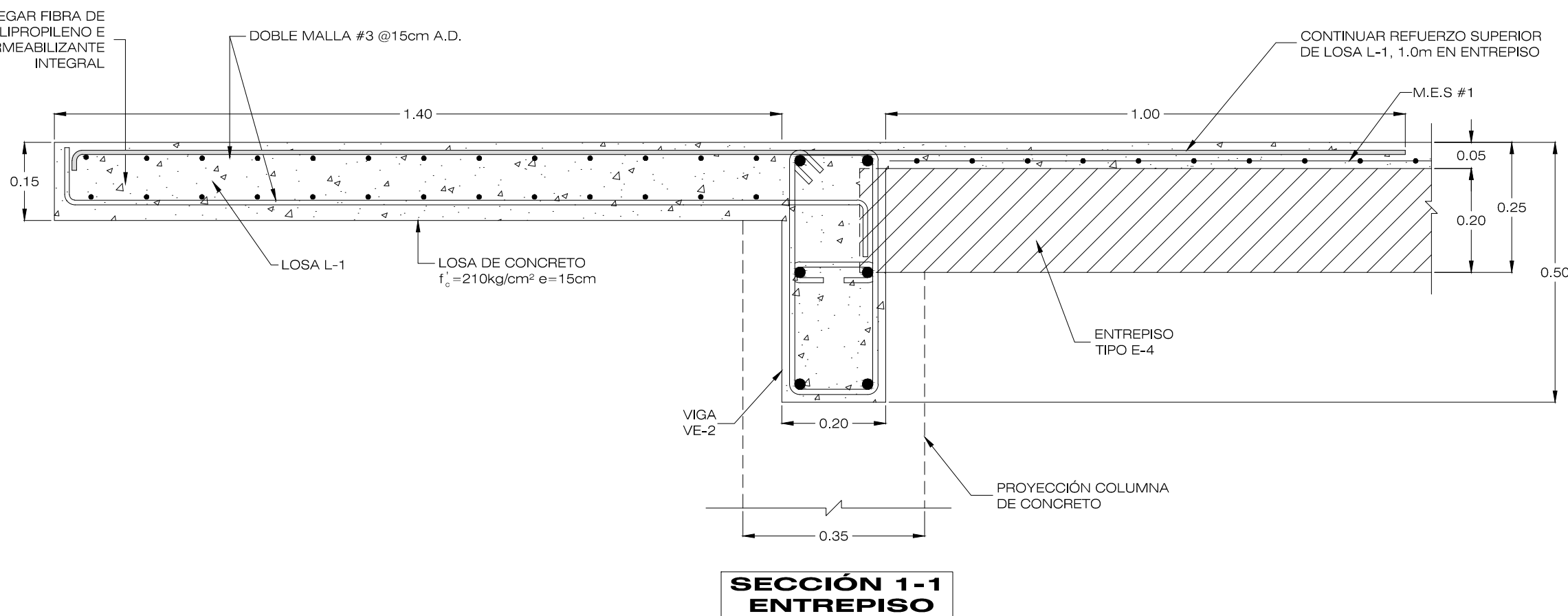
DET. DE SECCION ESCALA 1:10
