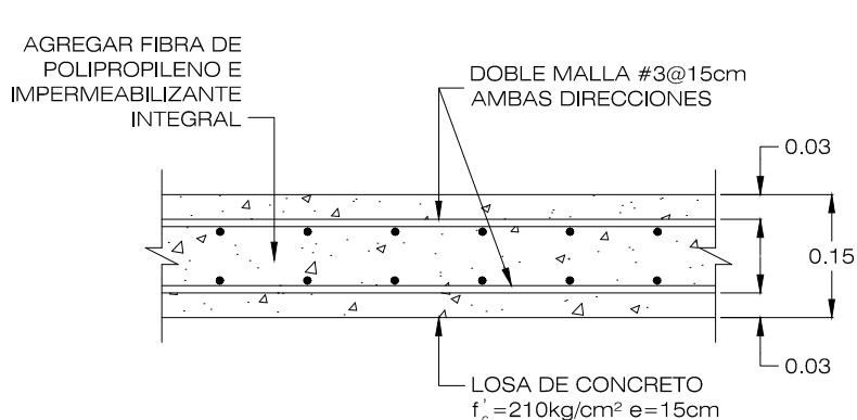
DET. DE LOSA ESCALA 1:10
