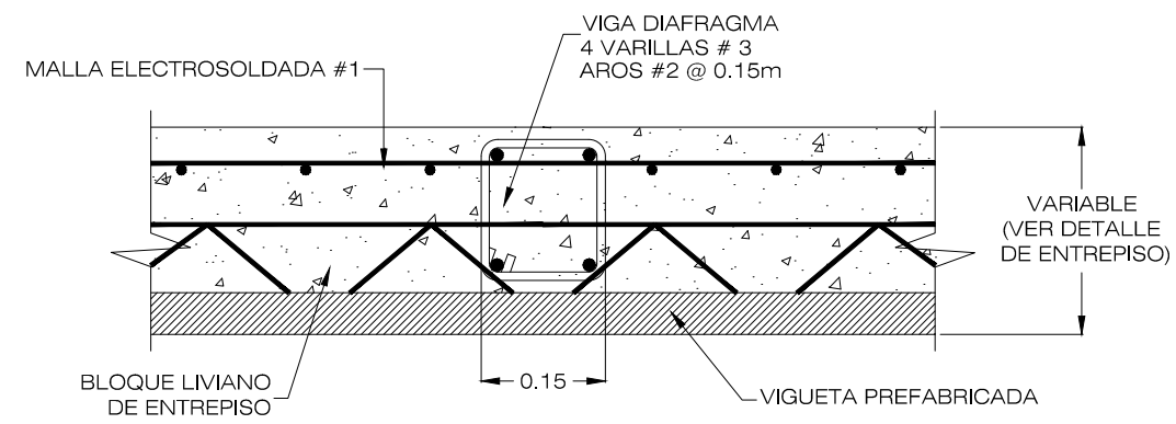
DET. VIGA DIAFRAGMA ESCALA 1:10
