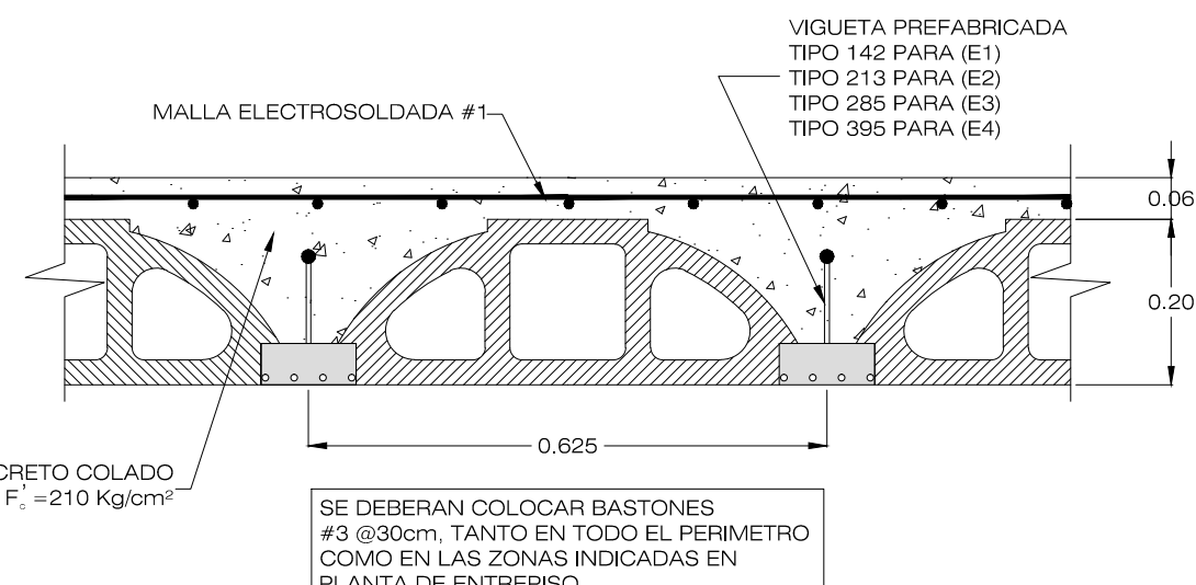
DET. DE ENTREPOSO ESCALA 1:10
