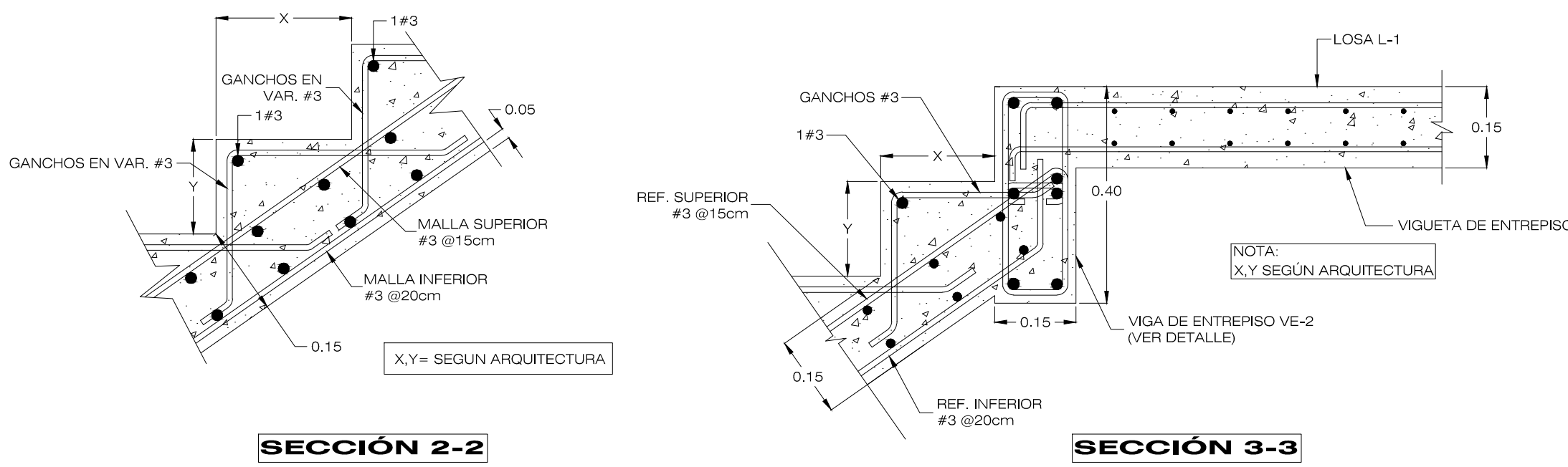
DETALLES SECCIONES DE ESCALERA ESCALA 1:10
