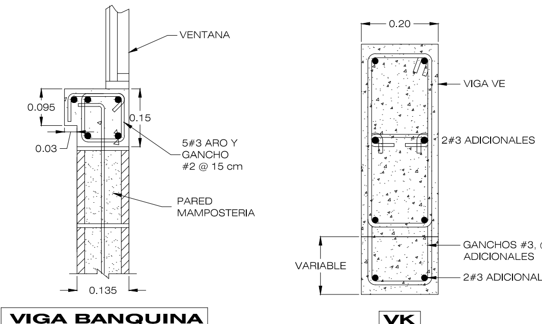
DETALLES DE VIGAS ESCALA 1:10
