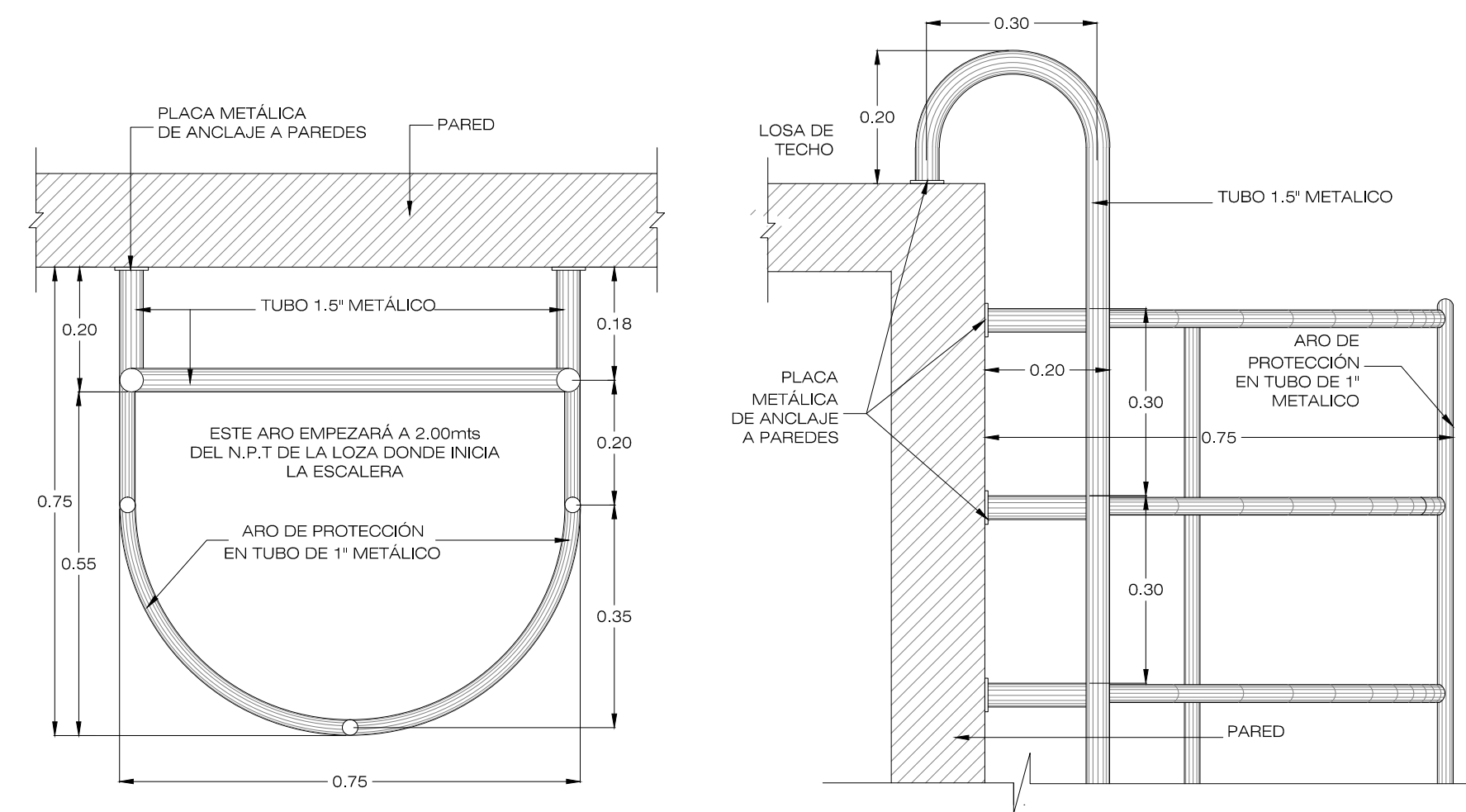
DET. ESCALERA TIPO MARINERA ESCALA 1:10
