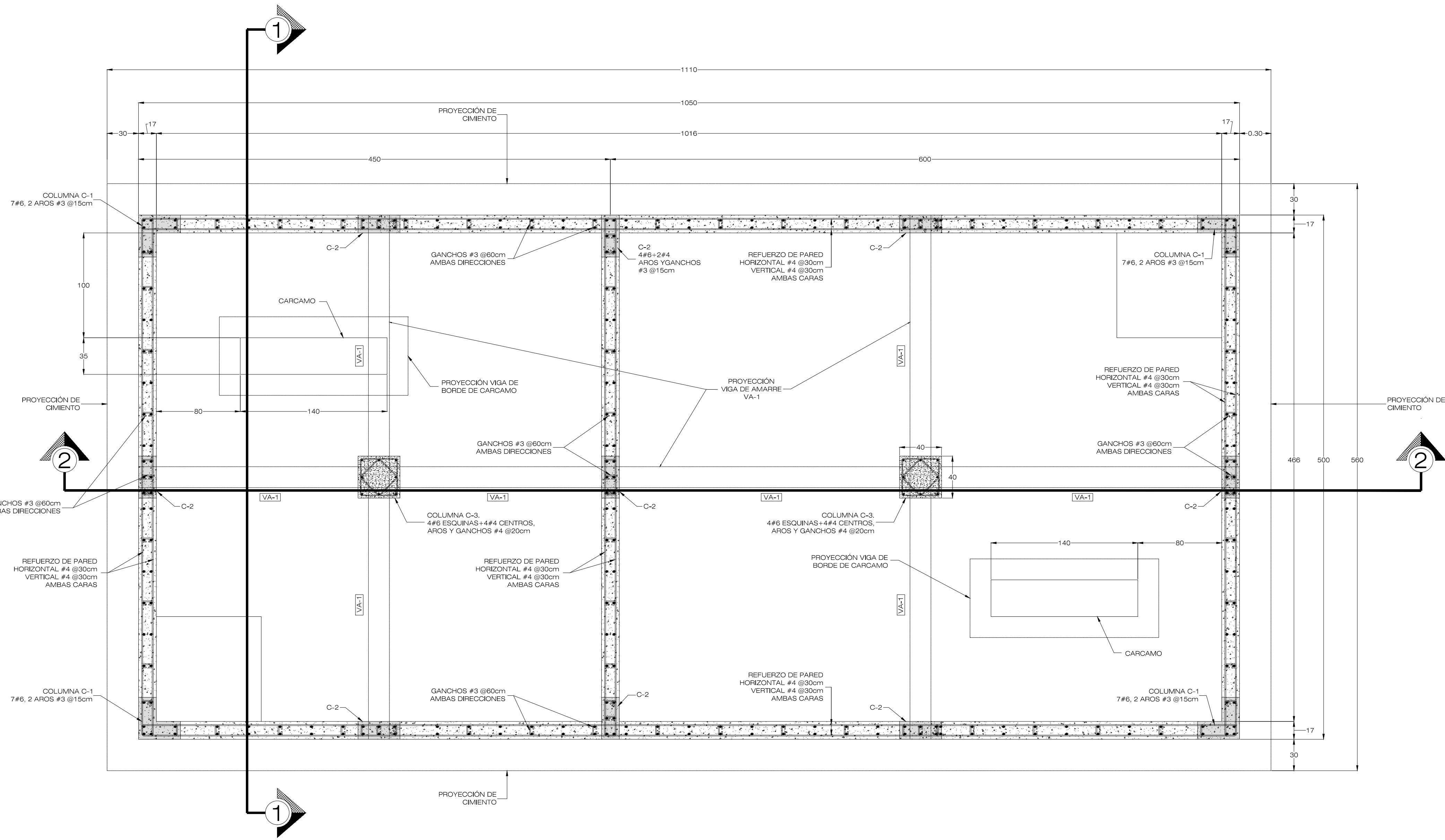
PLANTA DE CIMIENTOS TANQUE DE AGUA ESCALA 1:25
