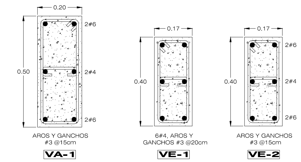
DETALLES DE VIGAS ESCALA 1:10
