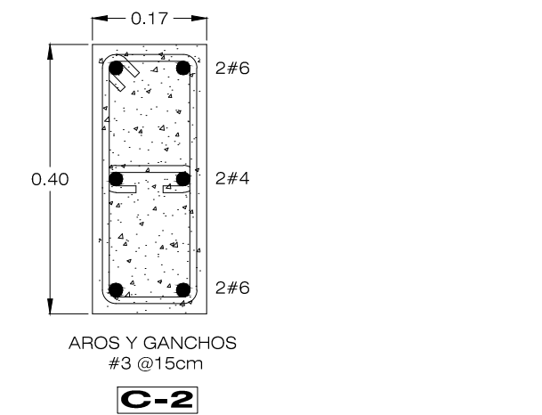
DETALLES DE COLUMNAS ESCALA 1:10
