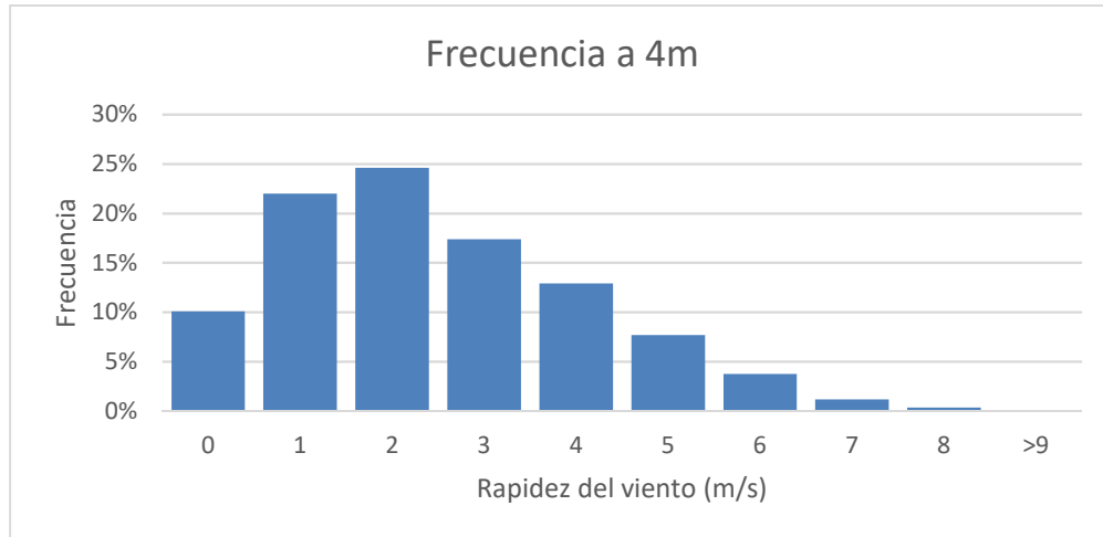
Figura 2. Frecuencia de la velocidad del viento a 4 metros.
