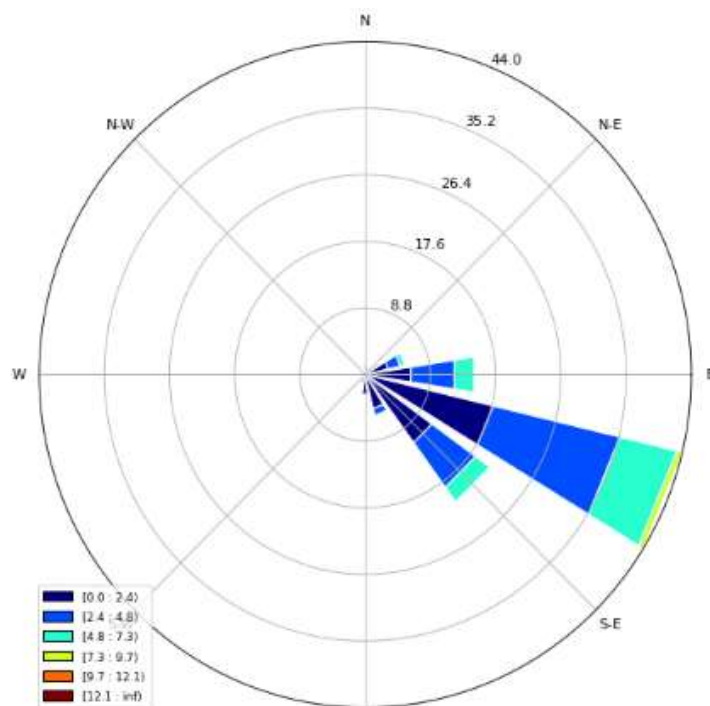
Figura 12. Rosa de los vientos a 12 metros de altura.
