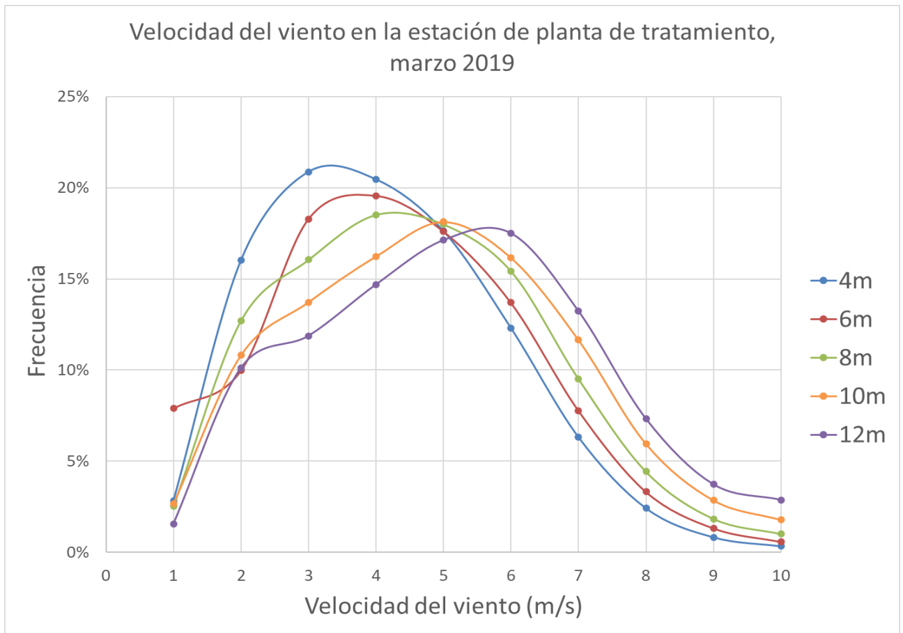
Figura 7. Velocidad del viento en la estación de planta de tratamiento, marzo 2019
