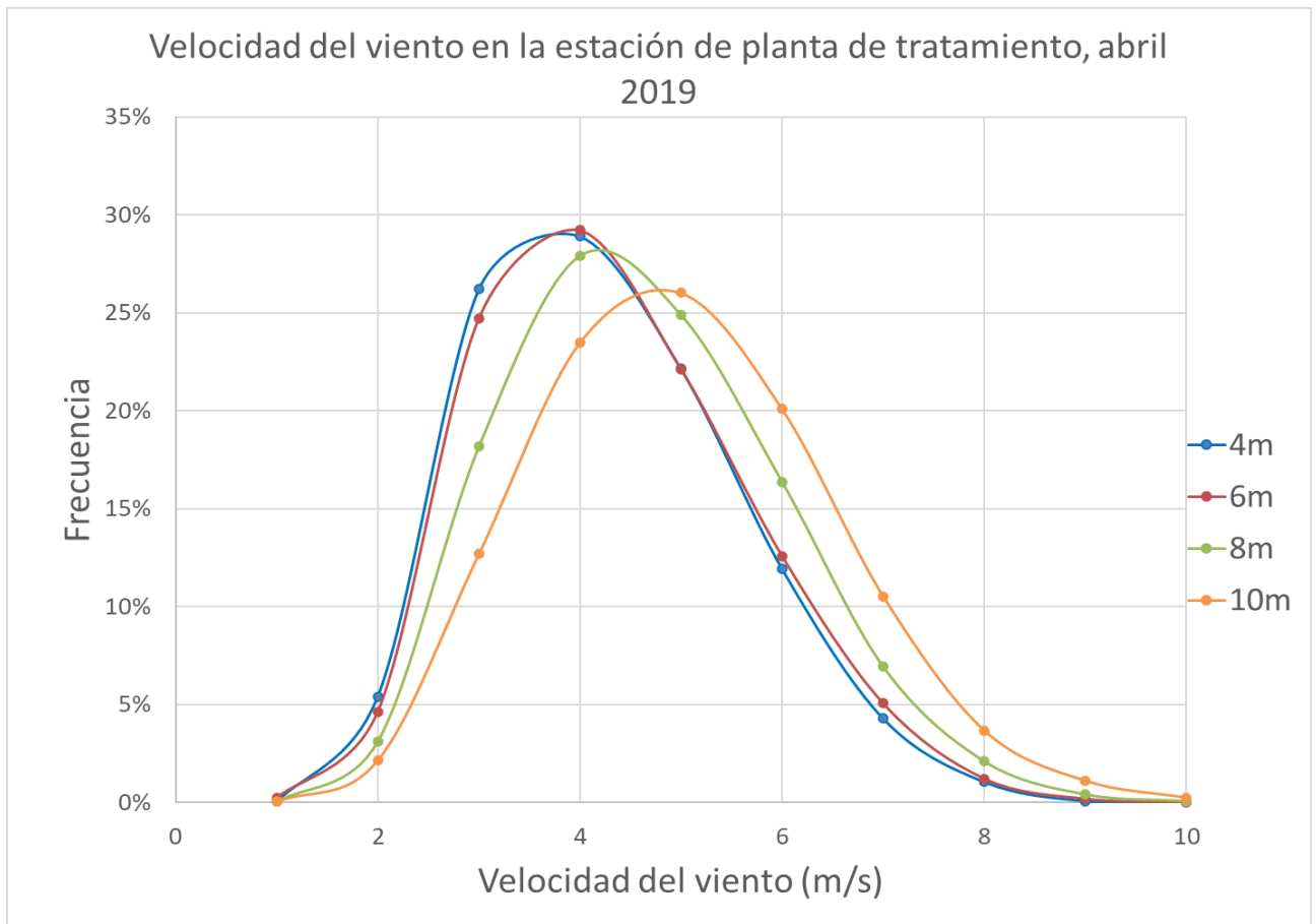
Figura 6. Velocidad del viento en la estación de planta de tratamiento, abril 2019
