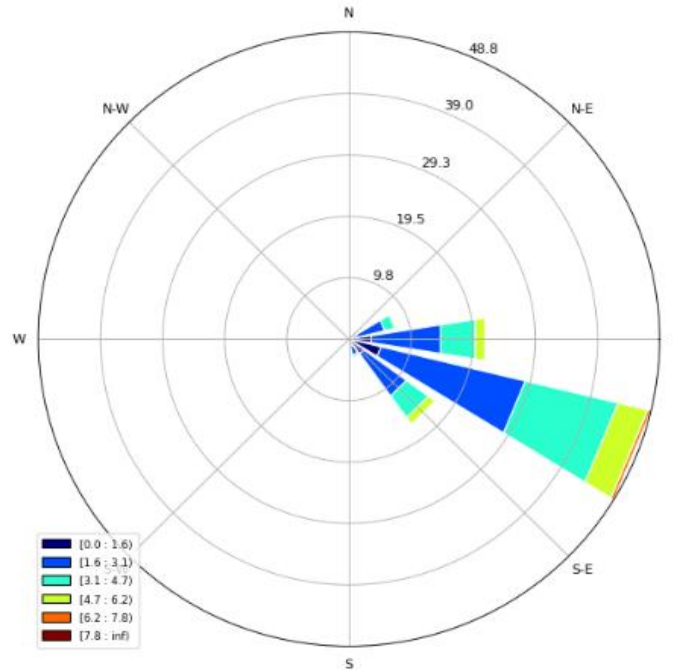
Figura 7. Rosa de los vientos a 4 metros de altura.
