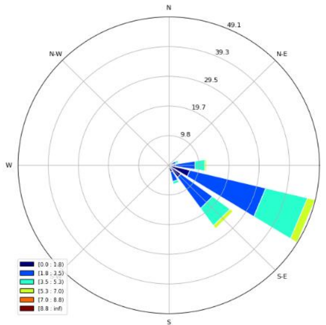
Figura 8. Rosa de los vientos a 6 metros de altura.
