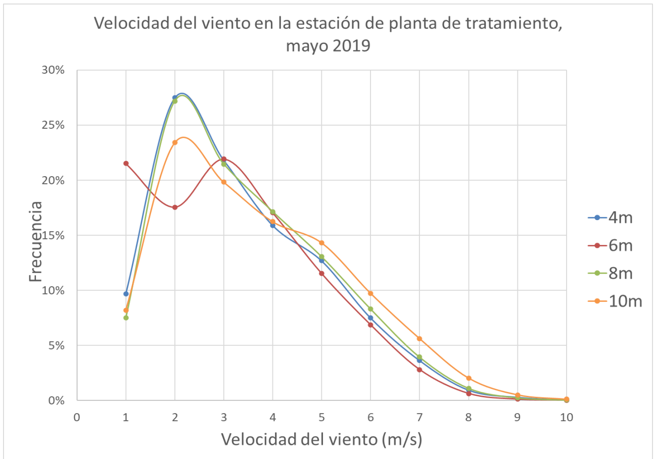
Figura 6. Velocidad del viento en la estación de planta de tratamiento, mayo 2019
