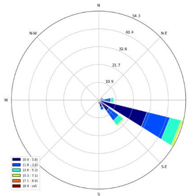
Figura 8. Rosa de los vientos a 6 metros de altura.
