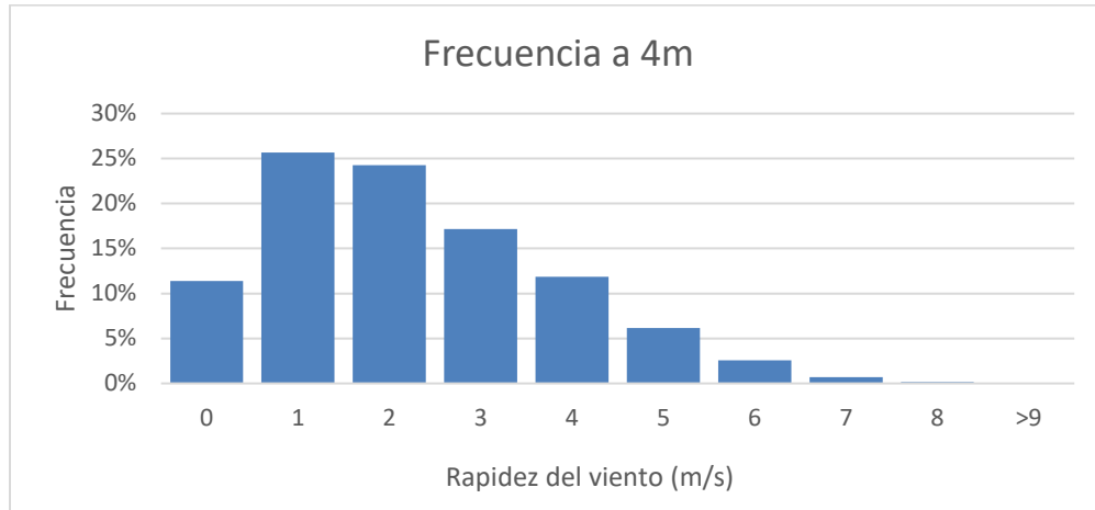
Figura 2. Frecuencia de la velocidad del viento a 4 metros.
