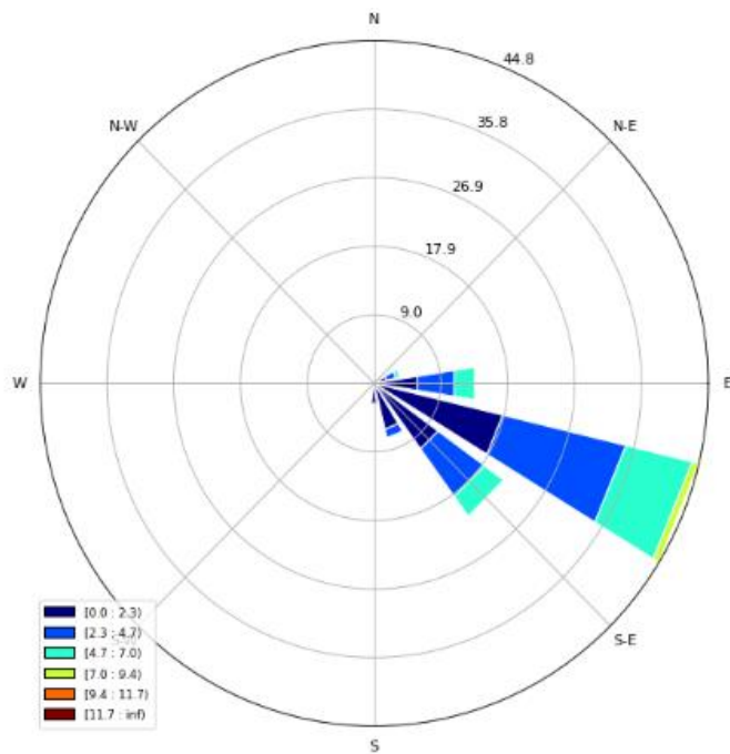
Figura 12. Rosa de los vientos a 12 metros de altura.
