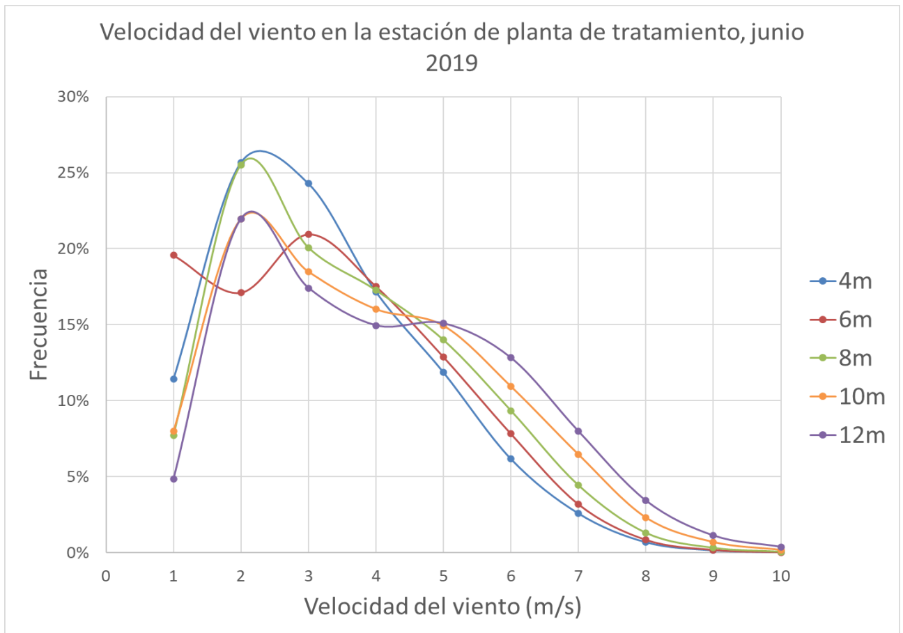
Figura 7. Velocidad del viento en la estación de planta de tratamiento, junio 2019
