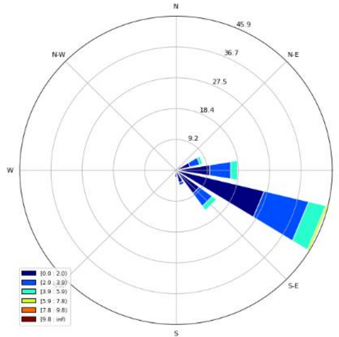
Figura 8. Rosa de los vientos a 4 metros de altura.
