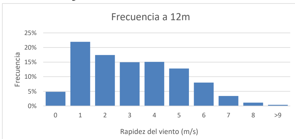
Figura 6. Frecuencia de la velocidad del viento a 12 metros.
