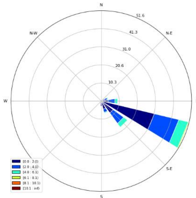
Figura 9. Rosa de los vientos a 6 metros de altura.
