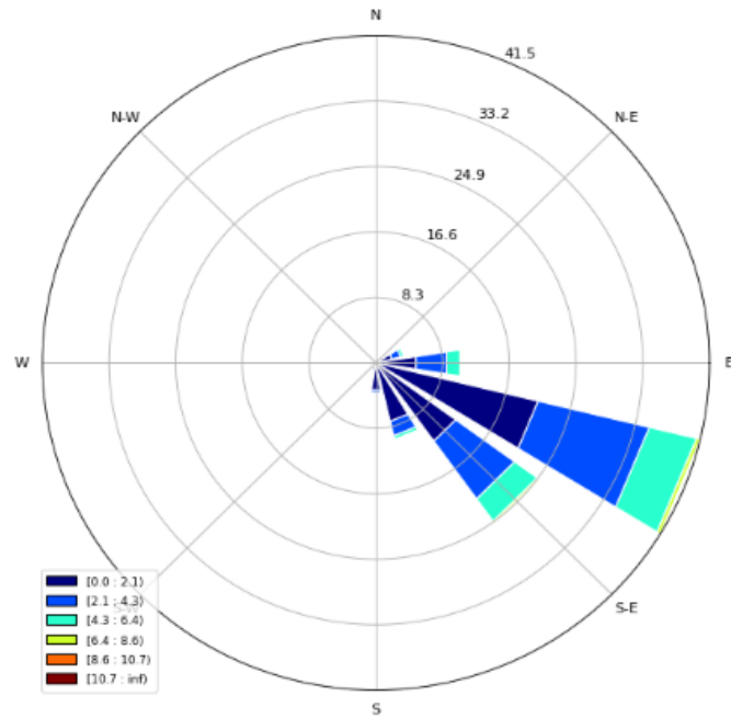
Figura 10. Rosa de los vientos a 8 metros de altura.
