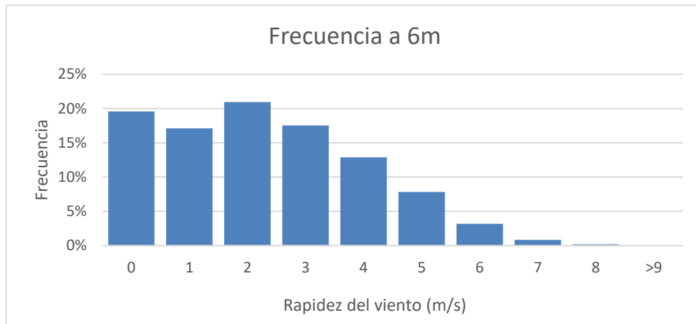
Figura 3. Frecuencia de la velocidad del viento a 6 metros.
