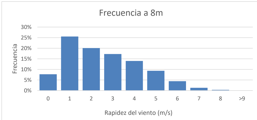
Figura 4. Frecuencia de la velocidad del viento a 8 metros.
