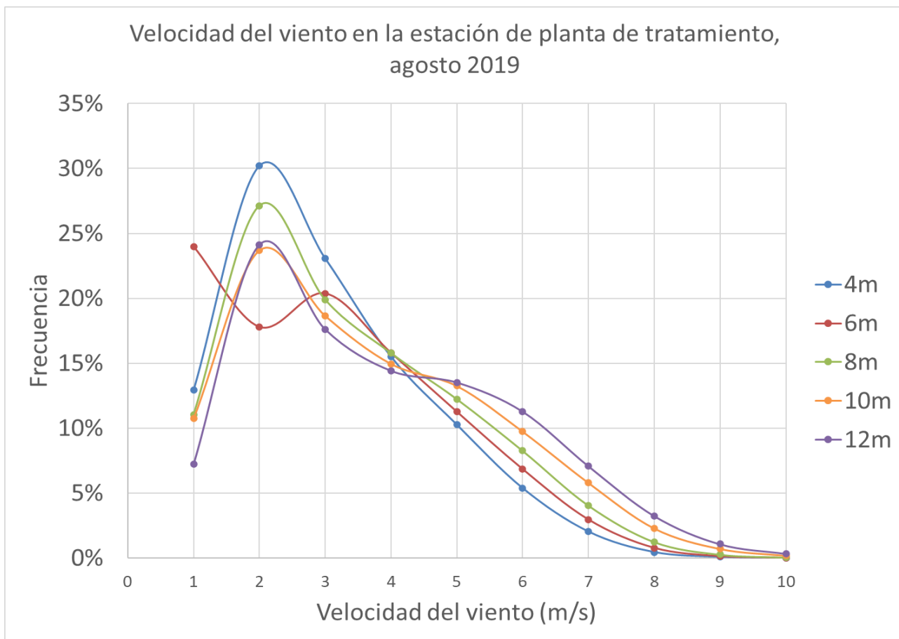
Figura 7. Velocidad del viento en la estación de planta de tratamiento, agosto 2019
