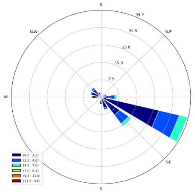
Figura 11. Rosa de los vientos a 10 metros de altura.
