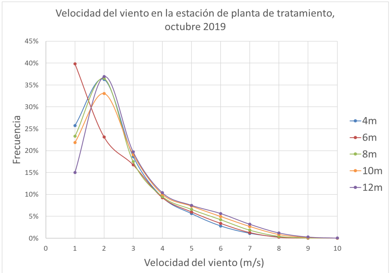
Figura 7. Velocidad del viento en la estación de planta de tratamiento, octubre 2019
