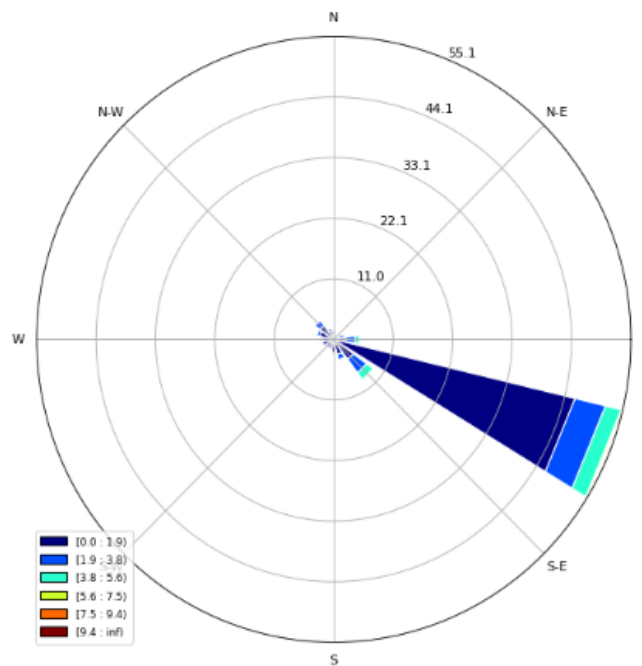
Figura 9. Rosa de los vientos a 6 metros de altura.
