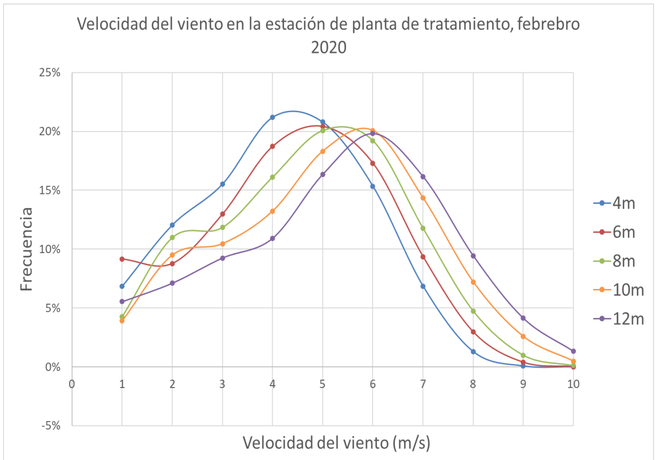
Figura 7. Velocidad del viento en la estación de planta de tratamiento, febrero 2020
