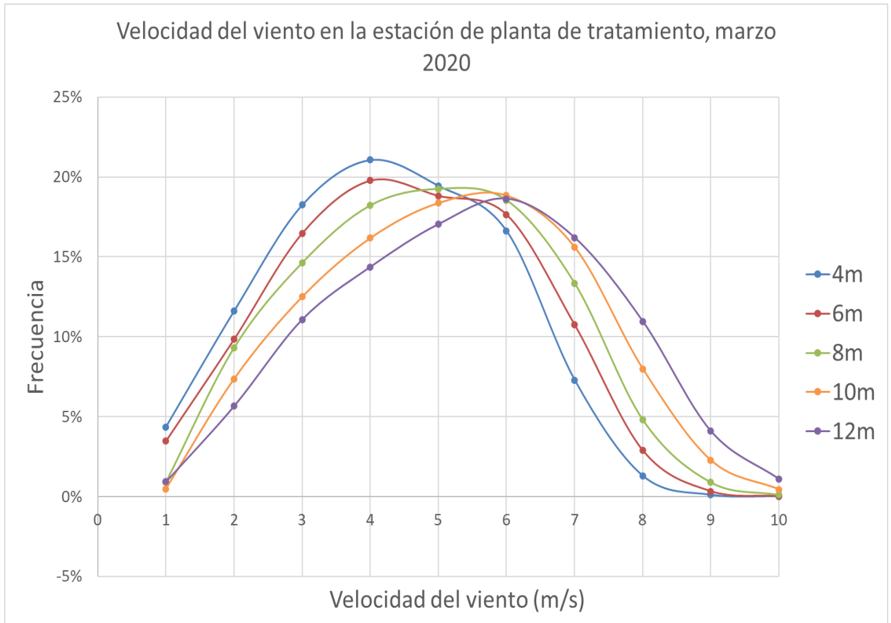
Figura 7. Velocidad del viento en la estación de planta de tratamiento, marzo 2020
