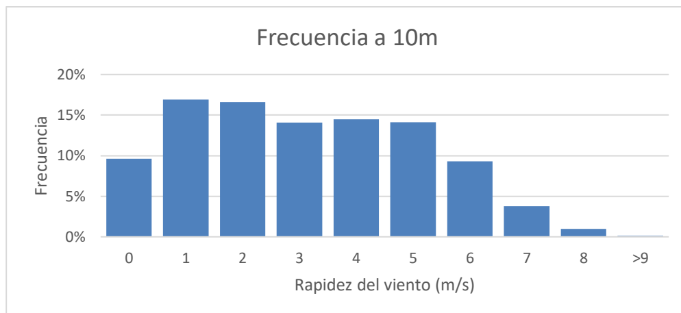
Figura 5. Frecuencia de la velocidad del viento a 10 metros.
