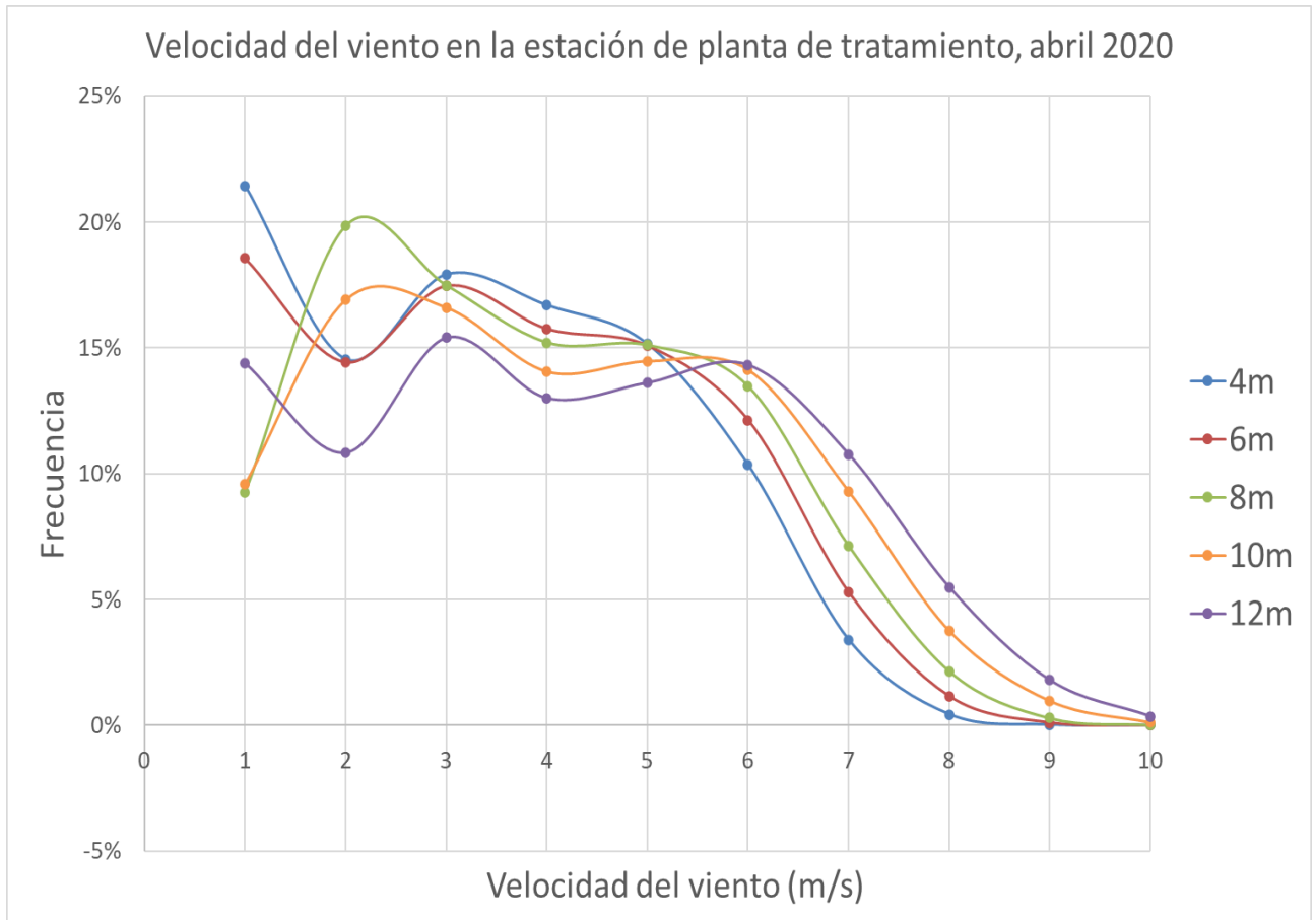
Figura 7. Velocidad del viento en la estación de planta de tratamiento, abril 2020
