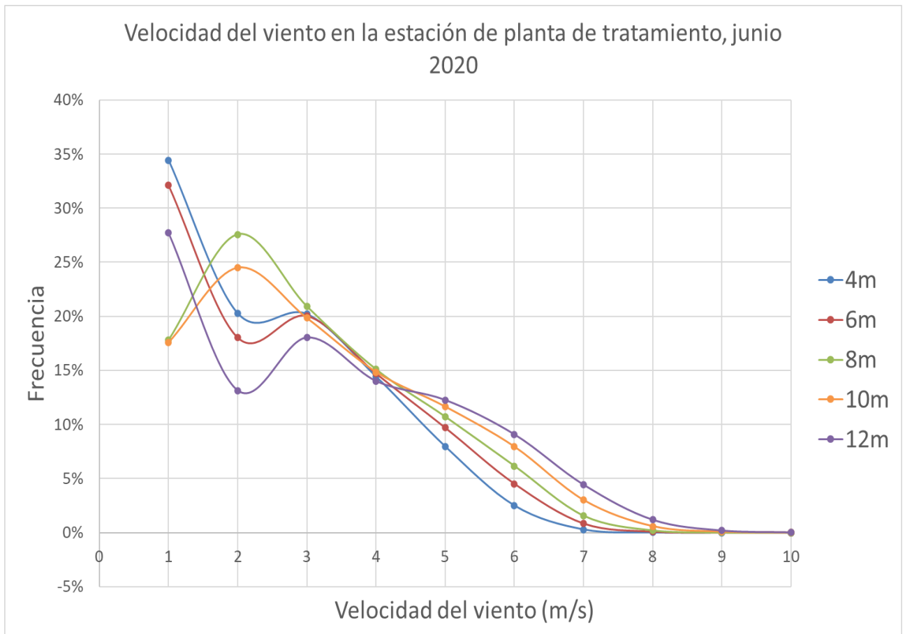
Figura 7. Velocidad del viento en la estación de planta de tratamiento, junio 2020
