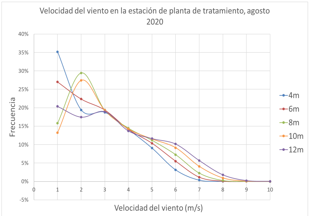
Figura 7. Velocidad del viento en la estación de planta de tratamiento, agosto 2020
