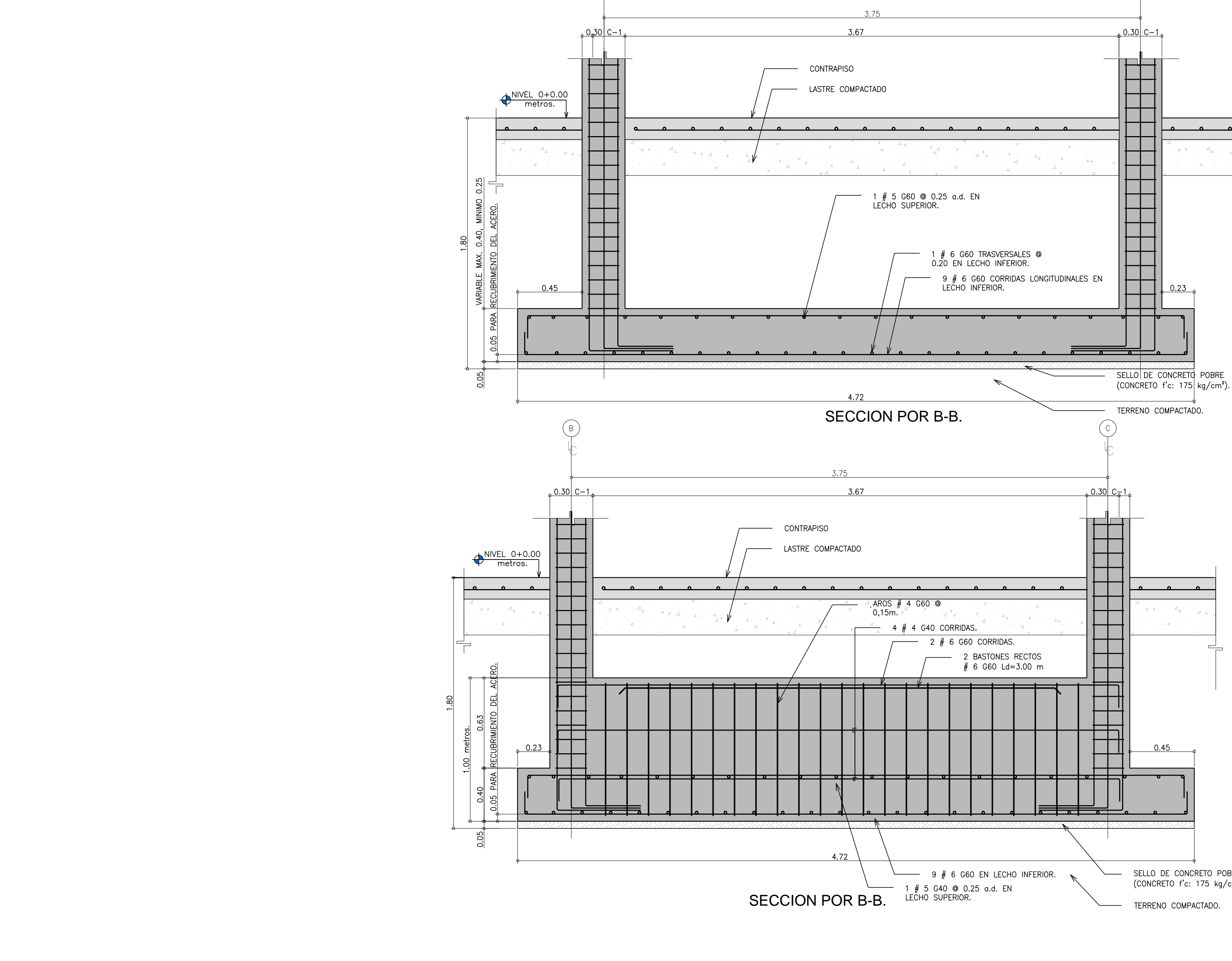
DETALLES DE PLACA TIPO PA-4.
