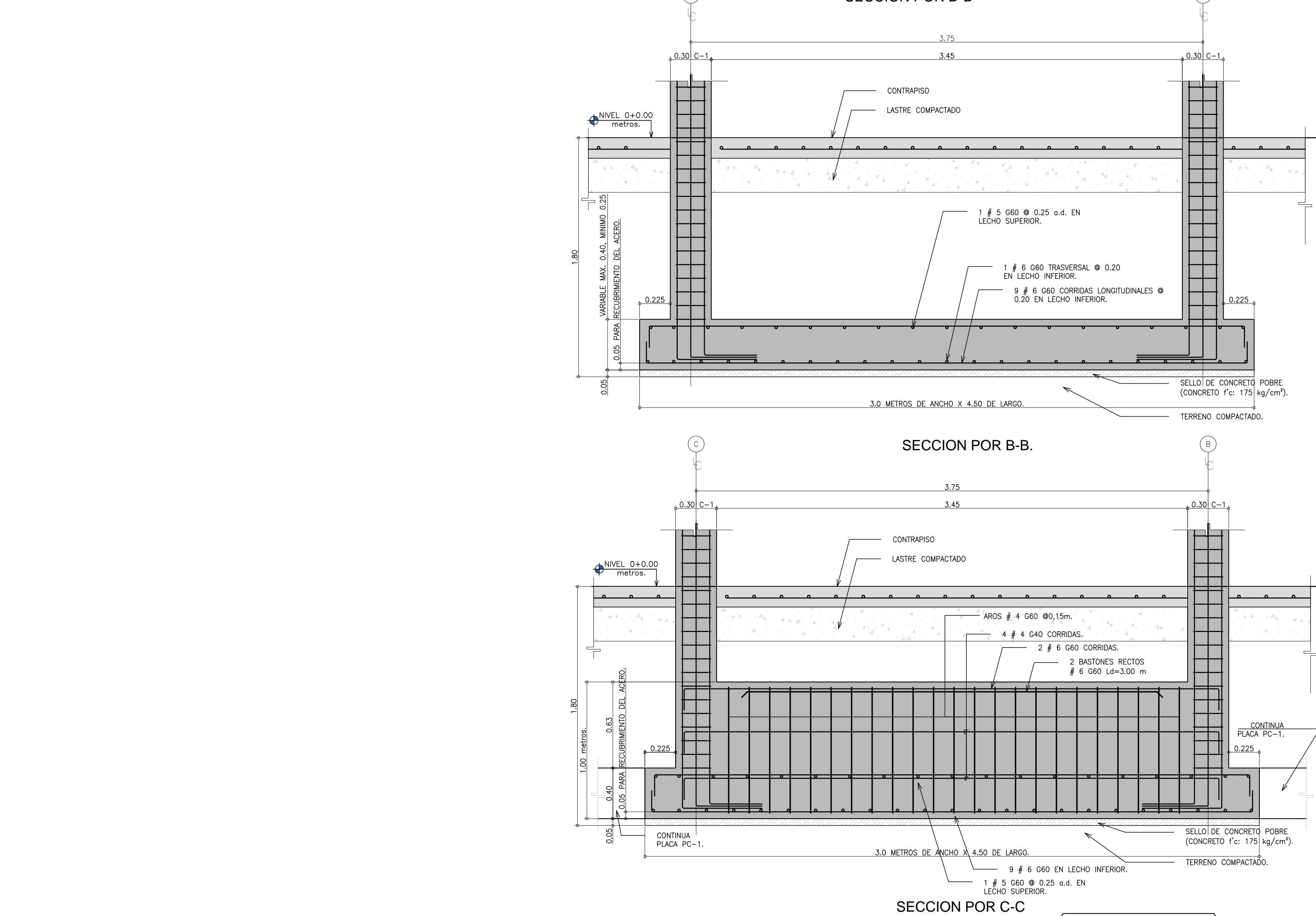
DETALLES DE PLACA TIPO PA-3.
