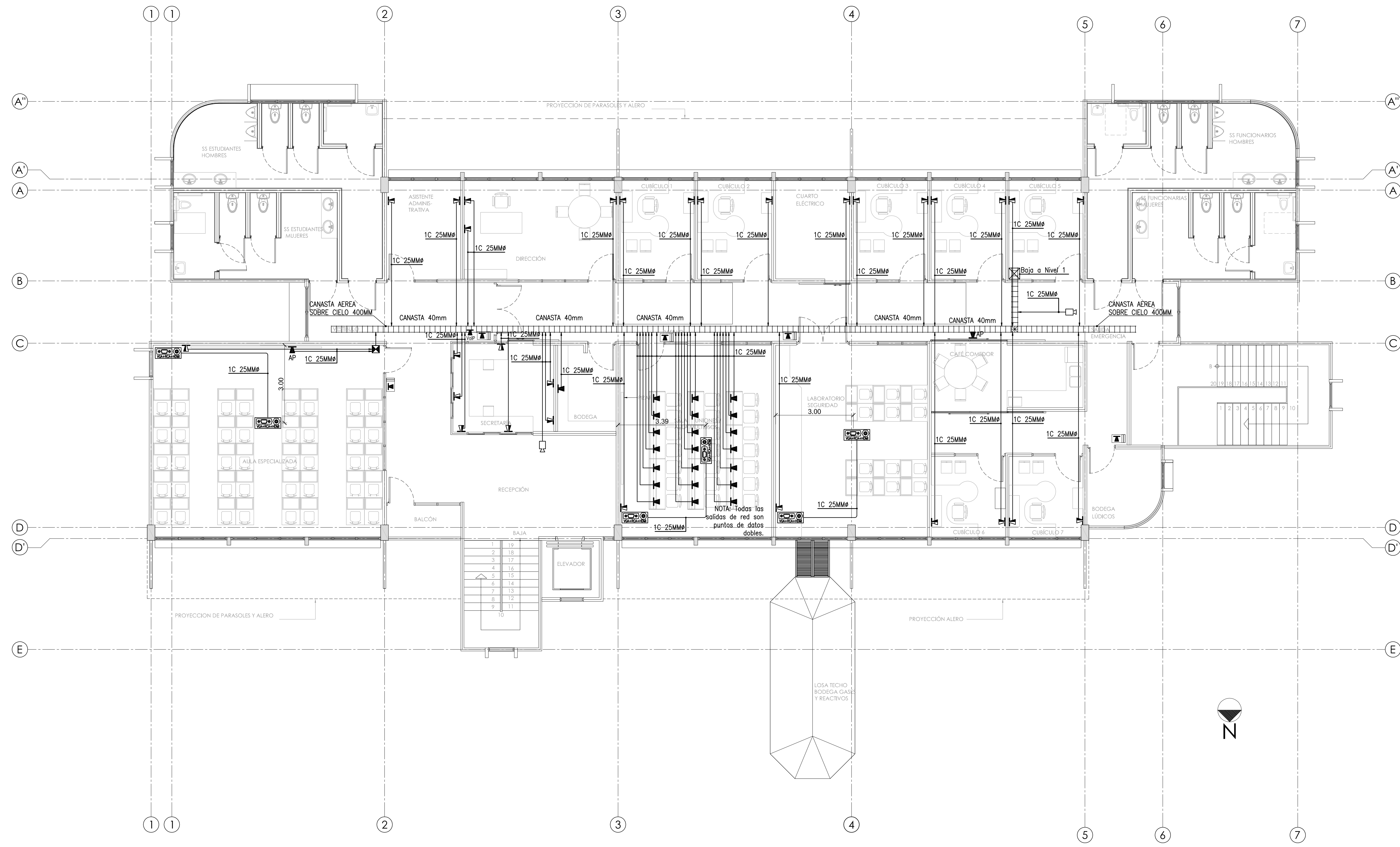
PLANTA DE DISTRIBUCIÓN DE CABLEADO ESTRUCTURADO SEGUNDO NIVEL ESCALA 1:75
